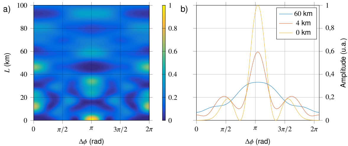
FIGURE 2.19 – Simulation de la figure d'interférence en fonction de la phase et de la propagation. La figure a) représente la déformation de la figure d'interférence en fonction de la propagation pour des taux de modulation a = b = 2.75 . Sur la figure b) sont représentées des coupes à 0 m, 4 km et 60 km.
