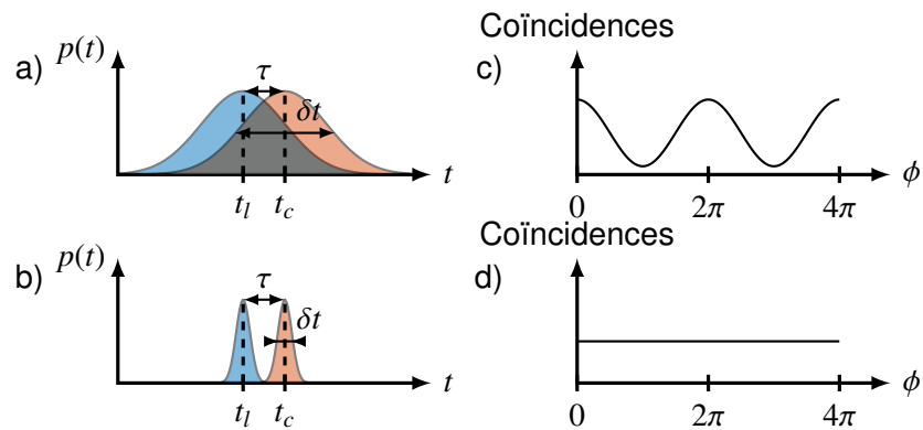
FIGURE 1.2 – Influence du recouvrement des chemins sur la figure d'interférence. Le moment d'émission d'un photon est connu avec une précision \delta t . Lorsque le photon entre dans un MZ dont le déséquilibre entre les bras vaut \tau la détection de ce photon en sortie du MZ peut conduire à l'observation d'une interférence. Le schéma a) représente le cas où \delta t > \tau , il y a un recouvrement des impulsions temporelles ayant suivi les deux chemins dans le MZ et on observe la figure d'interférence c) lorsqu'on déphase les deux bras du MZ. Le schéma b) représente le cas où les impulsions ne se recouvrent pas, \delta t \ll \tau , il n'y a plus d'interférence comme le montre le schéma d).
