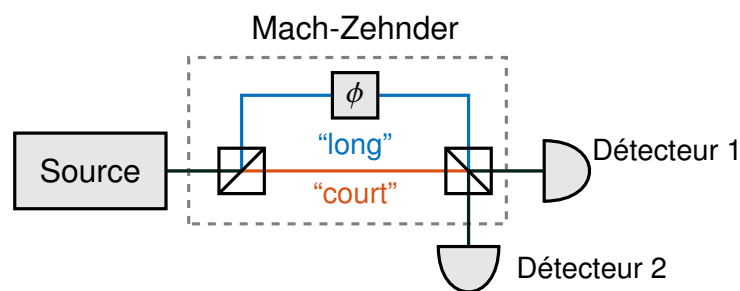
FIGURE 1.1 – Schéma d'interférences quantiques temporelles.
