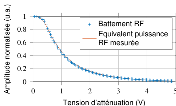
(f) Correspondance des amplitudes, Bob.
