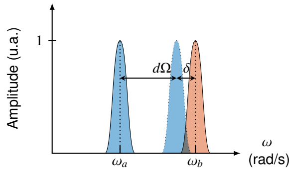
FIGURE 2.11 – Représentation de l'écart de fréquence entre les filtres. Le nombre d'entiers de fréquence de modulation, d , détermine l'ordre de l'interférence. Le reste, \delta , définit le taux de recouvrement des filtres contribuant à l'interférence.
