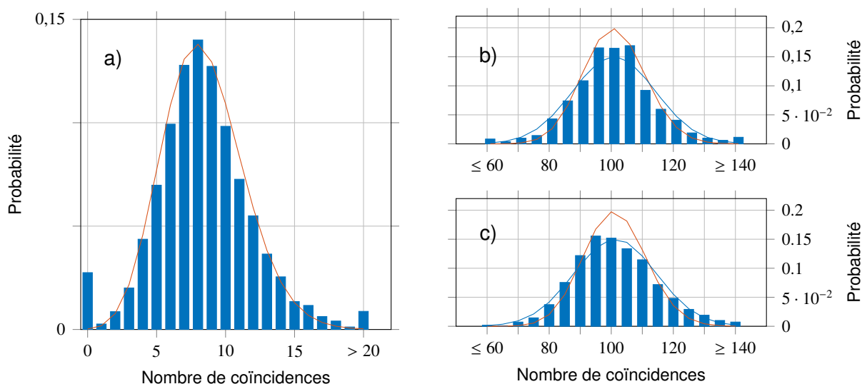
FIGURE 3.23 – Distribution du nombre de coïncidences par bin , pour des bins temporels de 65 ps en a) et 7, 8 ns en b) et c).
