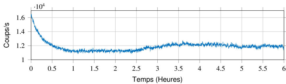
(a) Coups mesurés sur le détecteur 1.
