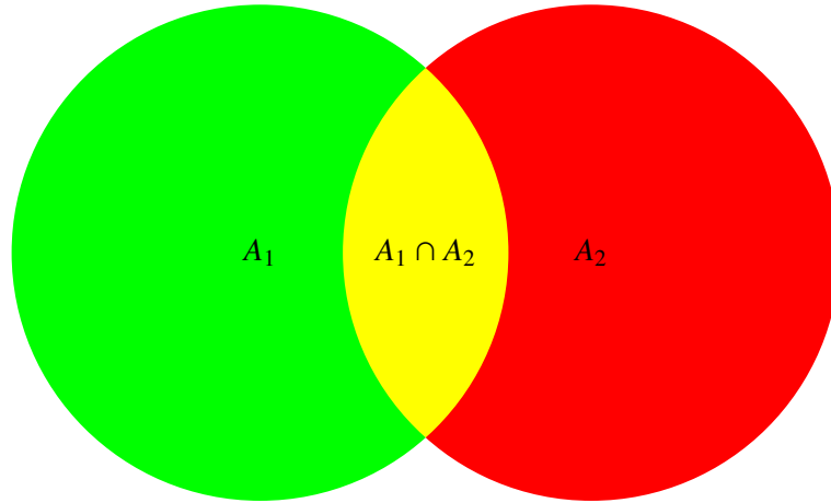
FIGURE A.2 – Représentation des événements correspondant à l'absorption du photon 1 ou 2.
