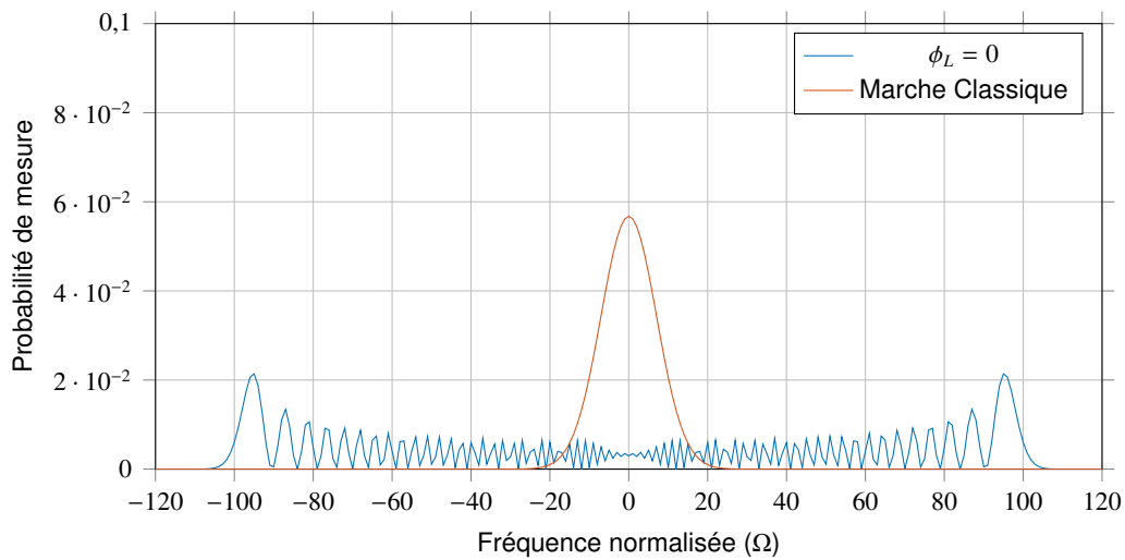
FIGURE 4.6 – Comparaison des distributions de probabilité après 100 pas, pour une marche aléatoire quantique en fréquence et son équivalent classique.
