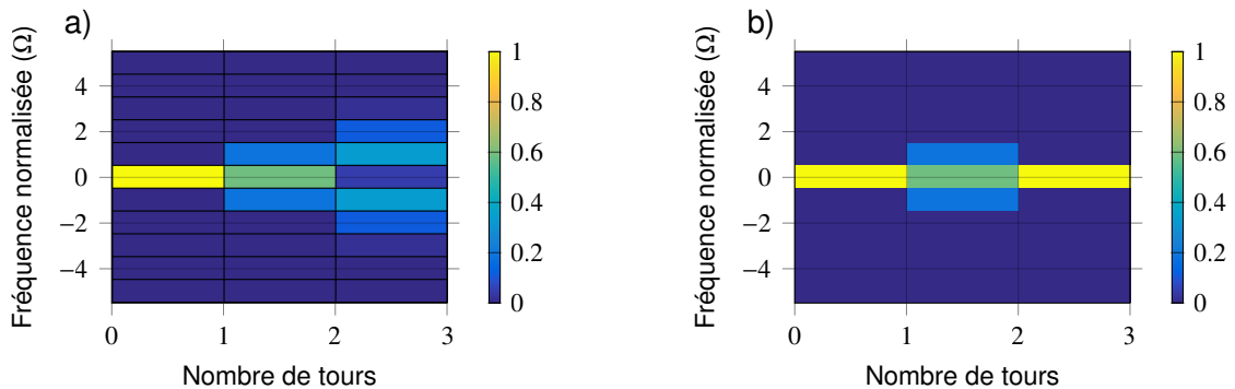
FIGURE 4.4 – Cas particuliers d'évolution d'une marche aléatoire. En a) est représenté l'évolution d'une marche avec une longueur de propagation tel que l'interférence, dans le modulateur, soit constructive, soit \phi_L = 0 . En b) est représenté le cas de l'interférence destructive, soit \phi_L = \pi .
