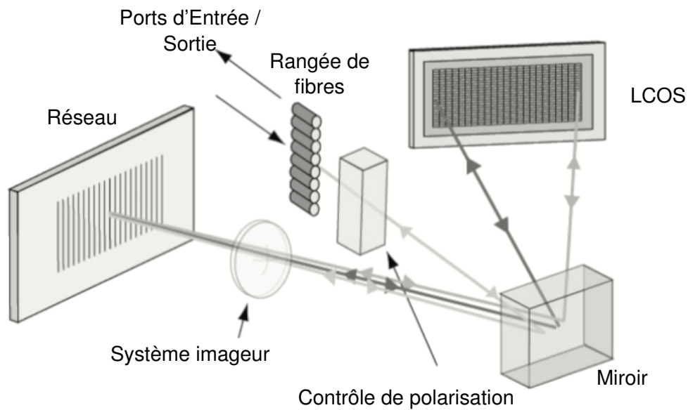
FIGURE 3.33 – Schéma du fonctionnement du WS4000s donné dans le manuel.
