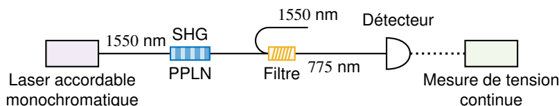
FIGURE 3.5 – Schéma de caractérisation de l'accord de phase du PPLN en SHG.
