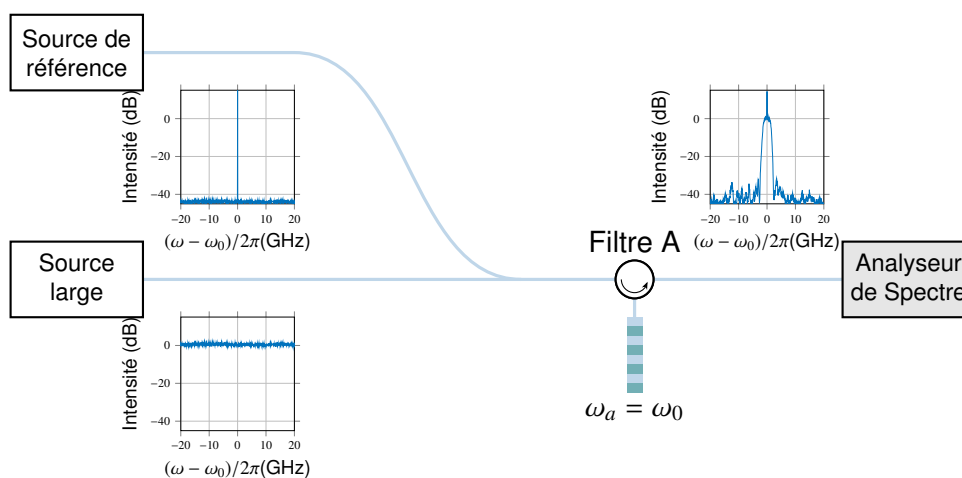
FIGURE 3.20 – Schéma de caractérisation de la stabilité du filtre A par rapport à un laser de référence.
