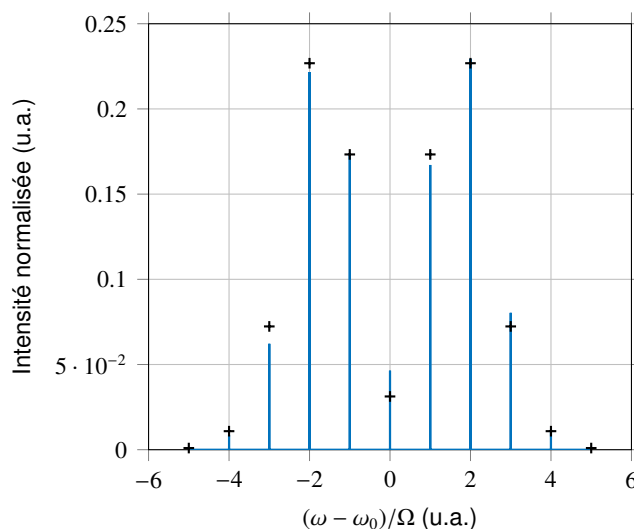
FIGURE 2.4 – Spectre en intensité mesuré en sortie de modulateur et normalisé par rapport à l'intensité totale. La courbe bleu représente les données expérimentales et les "+" noirs sont les valeurs théoriques correspondant à un taux de modulation de 2,78.
