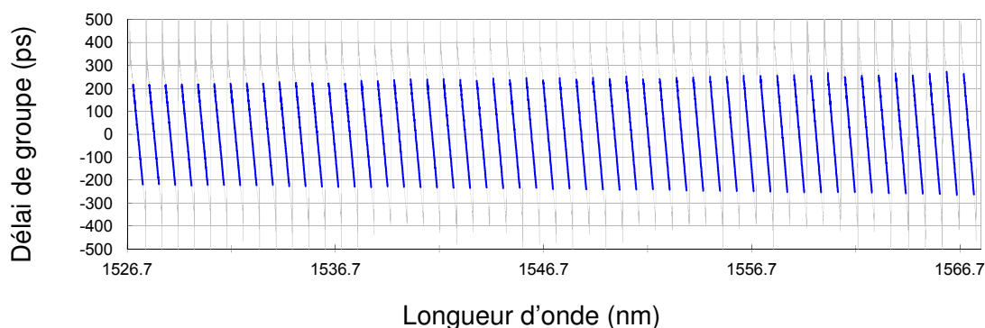
(b) Délai de groupe du MDCF.
