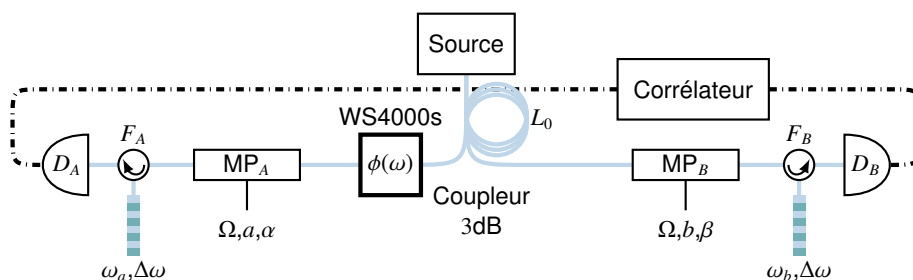
FIGURE 3.39 – Schéma expérimental de l'interférence à deux photons pour L_0 = 2 km.
