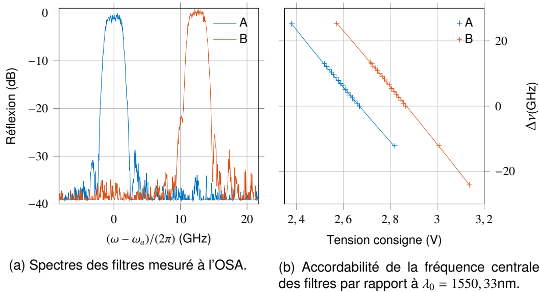
FIGURE 3.16 – Spectres des filtres et de la variation de leur fréquence centrale en fonction de la tension de consigne.
