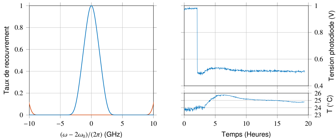
(a) Taux de recouvrement en fonction du décalage du second filtre.
