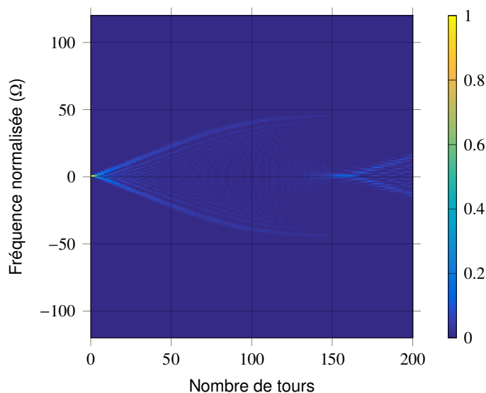
FIGURE 4.9 – Évolution d'une marche quantique en fréquence lorsqu'on tient compte de la dispersion et \phi_L = 0 .
