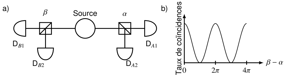
FIGURE 1.3 – Schéma de l'expérience de [Aspect et al., 1982b]. Des photons sont intriqués en polarisation et envoyés dans des systèmes de mesure dont on peut modifier indépendamment la base de mesure, via un paramètre \alpha ou \beta , comme représenté sur le schéma a). La probabilité de mesurer les photons intriqués dépend alors uniquement de \beta - \alpha , dont l'évolution est représentée schéma b).
