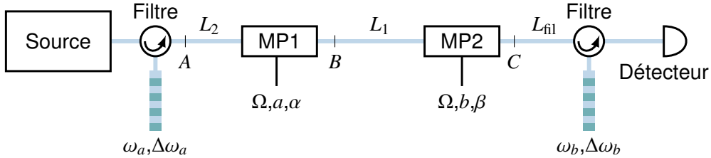
FIGURE 2.10 – Schéma de l'interférence à un photon en fréquence.
