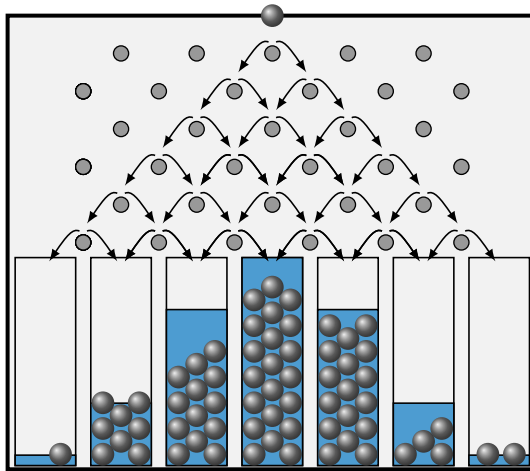
FIGURE 4.1 – Schéma d'une planche de Galton. Une bille chute le long d'une planche cloutée et possède une probabilité équivalente d'aller à gauche ou à droite de chaque clou. En bas de cette planche est représenté le résultat de l'expérience renouvelée un grand nombre de fois. Le niveau de bleuté correspond à la loi binomiale vers laquelle tend cette distribution.
