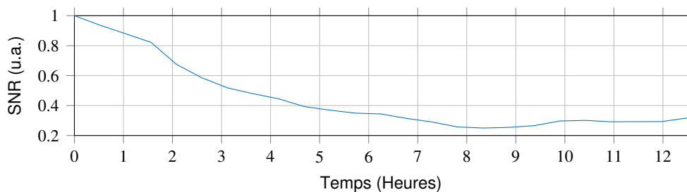
(c) Rapport signal sur bruit par pic de coïncidences (30 min par pic).
