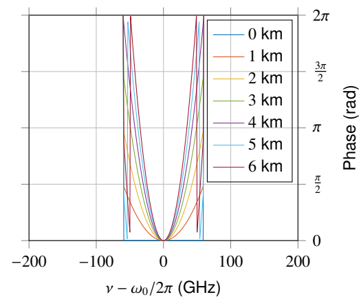
FIGURE 3.35 – Spectre en phase appliqué au WS4000s en fonction de la distance.
