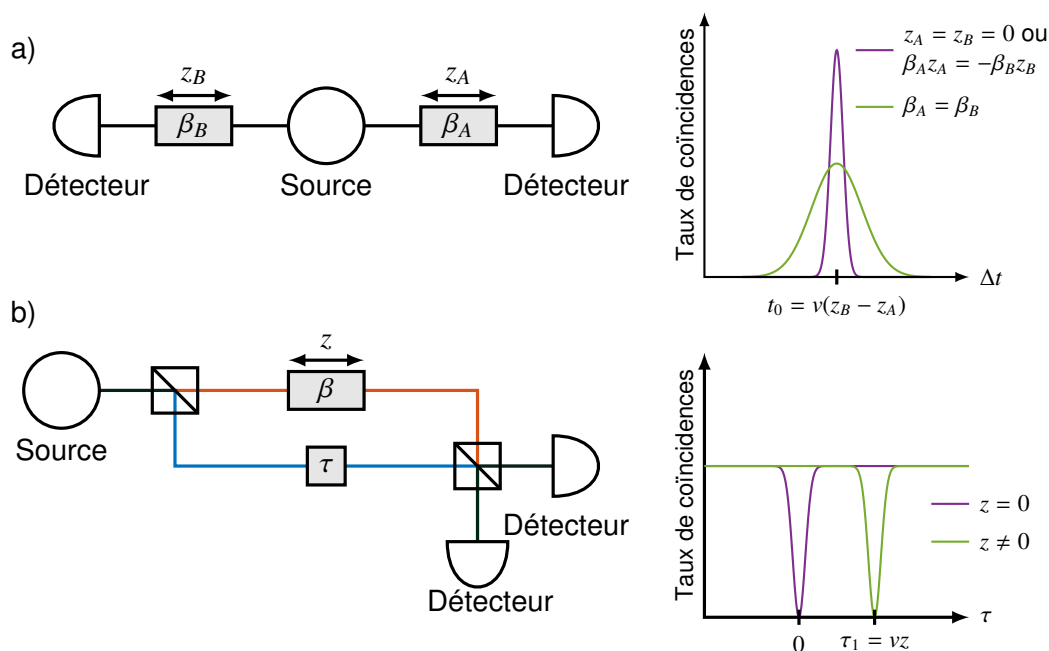
FIGURE 1.6 – Schémas de compensation de dispersion. Dans les deux cas, la source émet des photons intriqués en temps-fréquence et on mesure les coïncidences entre ces photons. Le schéma a) représente la compensation non-locale de dispersion introduite par [Franson, 1992]. On observe un pic de coïncidence lorsqu'on représente le nombre de photons mesuré en fonction de la différence de temps d'arrivée sur les détecteurs. On observe un étalement du pic de coïncidences lorsque les photons sont dispersés, cet exemple est légendé \beta_A = \beta_B . Lorsque les dispersions se compensent, \beta_A z_A = \beta_B z_B , on retrouve la largeur du pic de coïncidence sans dispersion. Le schéma b) représente l'auto-compensation de dispersion introduite par [Steinberg et al., 1992a]. On observe une chute des coïncidences, appelée dip , lorsque le retard \tau entre les deux bras tend vers 0 (effet HOM). La largeur du dip est une signature du degré de cohérence entre les photons observés. Lorsque qu'on introduit un milieu dispersif \beta de longueur z sur un des bras, [Steinberg et al., 1992a] montre que la largeur du dip n'est pas affectée par l'étalement de l'enveloppe temporel du photon dispersé. Il attribue cet effet à la relation de fréquence existant entre les photons intriqués et mesurés en coïncidence.
