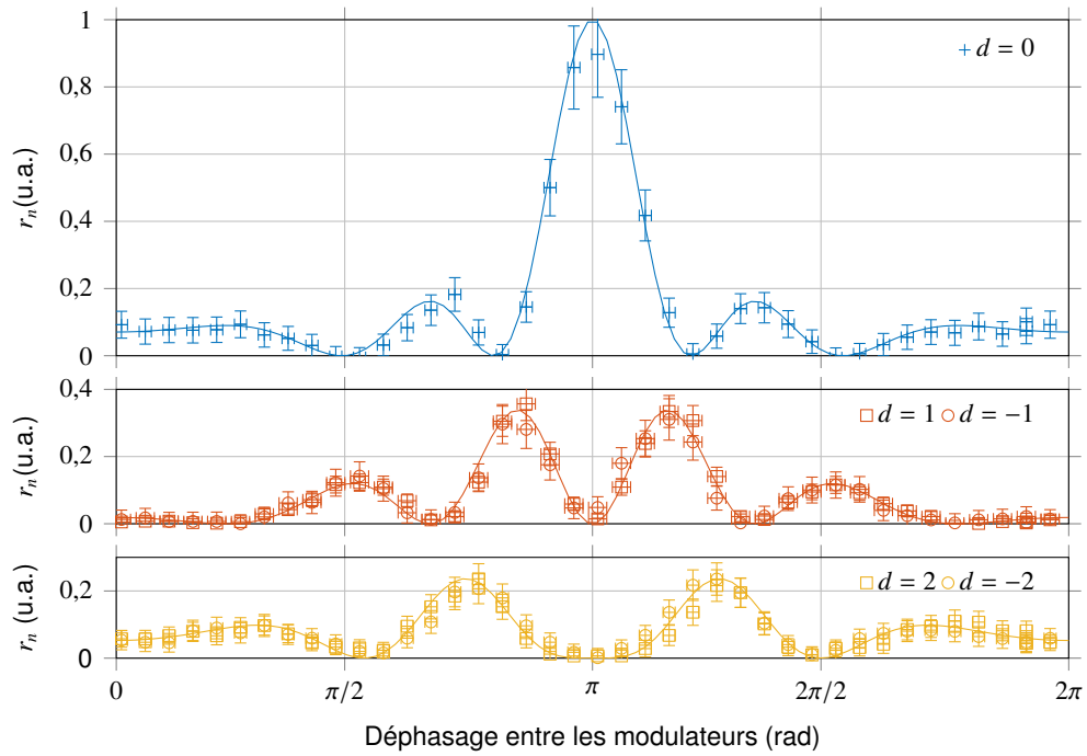
FIGURE 3.32 – Interférence à deux photons.
