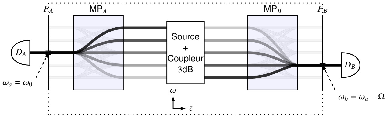
FIGURE 2.14 – Schéma d'interférence à deux photons avec propagation.
