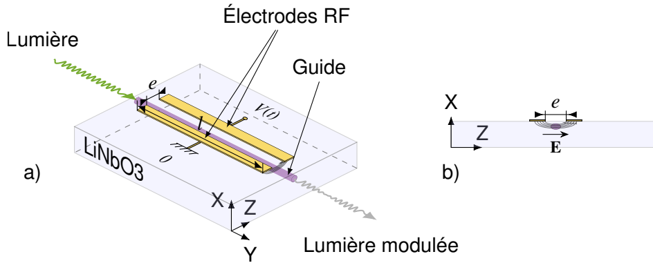
FIGURE 2.2 – Schéma d'un modulateur de phase en coupe X. La figure a) montre que la disposition des électrodes induit la génération d'un champ électrique orienté selon l'axe cristallin Z dans le guide. Comme le montre la figure b), cette orientation permet de bénéficier d'une modulation d'indice, proportionnelle au plus grand coefficient du tenseur de permittivité diélectrique du cristal ( r_{33} ), pour une onde optique polarisée suivant l'axe Z.
