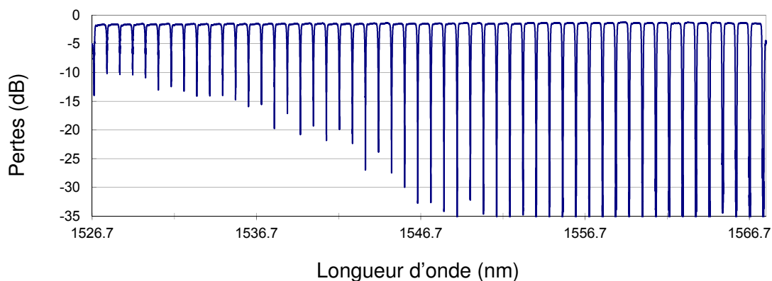
(a) Pertes d'insertion du MDCF en fonction de la longueur d'onde.
