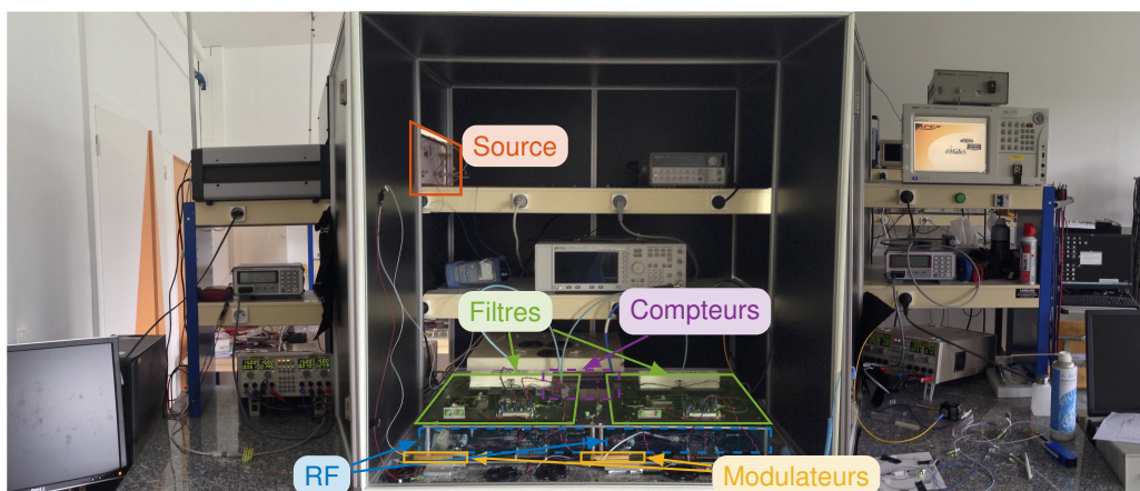
FIGURE 3.31 – Photographie du dispositif expérimental.
