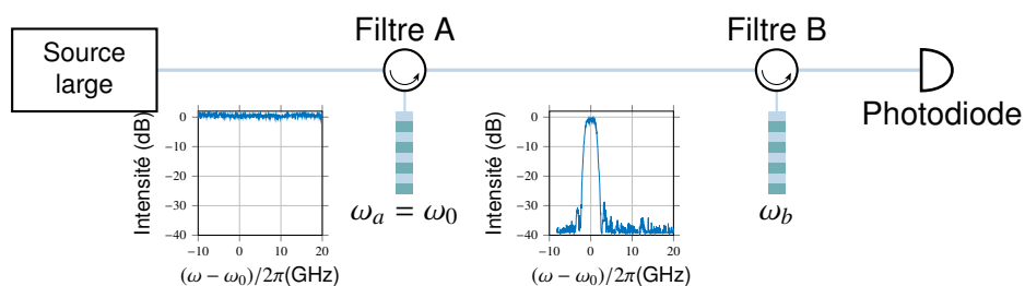
FIGURE 3.17 – Schéma de caractérisation de la stabilité relative des filtres.
