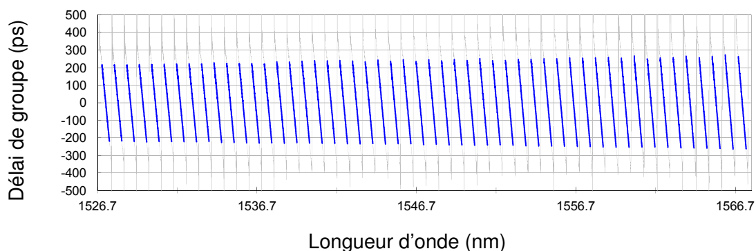
(b) Délai de groupe du MDCF.
