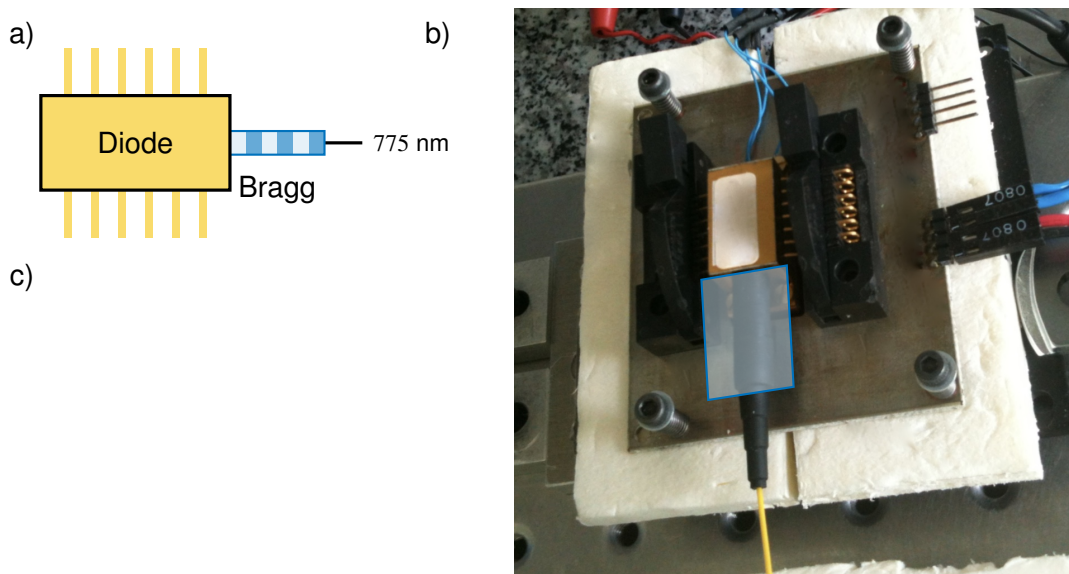
FIGURE 3.2 – Présentation de la diode laser de pompe. En a) est représenté un schéma de la diode laser, et en b) une photographie. Nous avons rappelé la position du filtre de Bragg à l'aide d'un encadré bleu sur le schéma b). Le graphique c) représente le spectre mesuré de cette diode, pour une température de 28°C et un courant d'alimentation de 53 mA.
