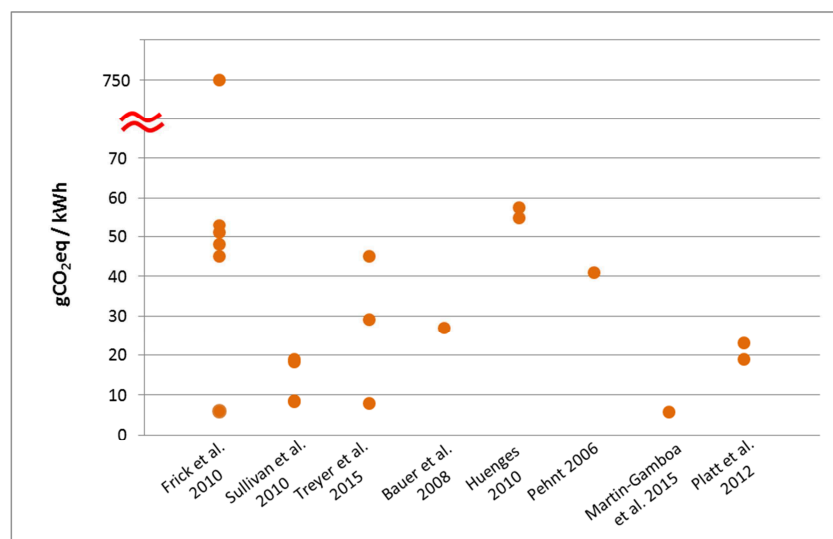
Figure i. ACV des EGS : revue de littérature (résultats d'émissions de GES)
