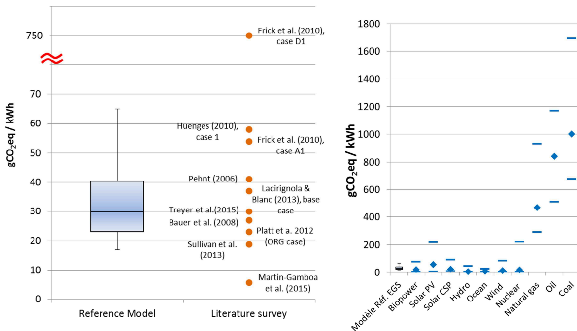
Figure v. Profil environnemental de la filière EGS en Europe centrale, comparé avec des ACV d'EGS de la littérature (à gauche) et avec des ACV d'autres technologies énergétiques (Moomaw et al. 2011)
