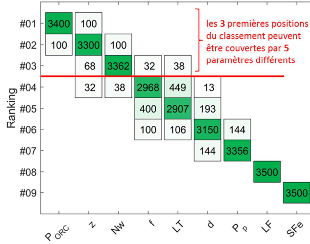
Figure viii. Résultats agrégés des 3500 GSA
