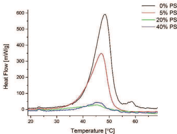
Figure 10 Thermogrammes normalisés des différentes micelles obtenus par calorimétrie différentielle à balayage. Les micelles contenant une plus grande quantité d'homopolymère montrent une décroissance de la contribution cristalline du PEO.
