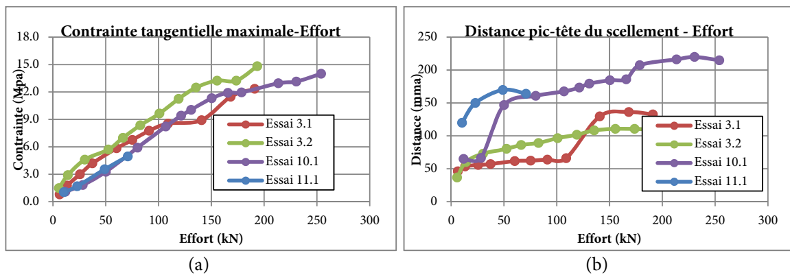
Figure 246 Influence du diamètre de forage sur le pic des contraintes tangentielles (a) Valeur (b) Distance pic-tête du scellement en fonction de l'effort en tête du scellement ( d_b = 25\text{mm} ; d_g = 64\text{mm} )
