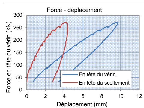
Figure 400 Courbe de comportement: force en fonction du déplacement en tête du vérin et en tête du scellement
