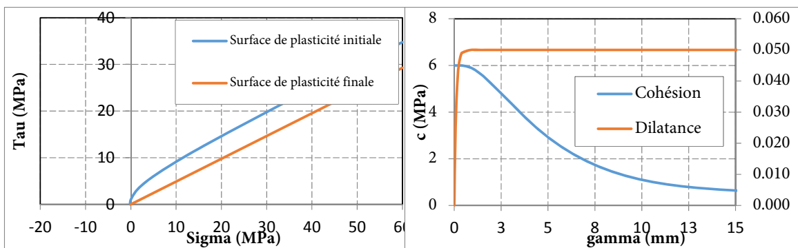
Figure 110 Illustration du modèle de comportement de l'interface barre-scellement (a) surfaces de plasticité (b) fonctions de la cohésion et de la dilatace
