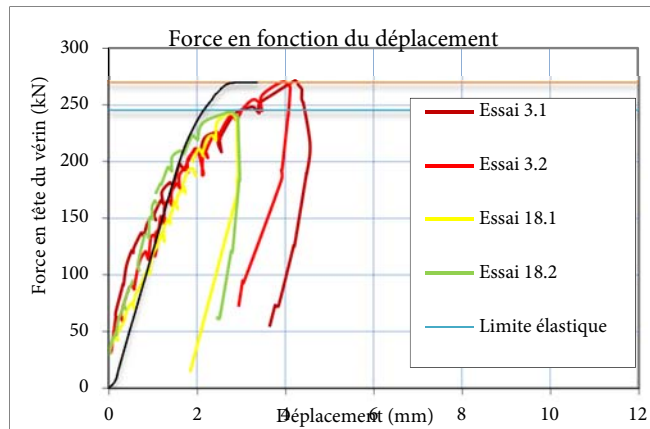
Figure 256 Influence de la canule d'injection sur la courbe de comportement: effort axial - déplacement en tête du scellement calculé à partir des capteurs LDT ( d_b = 25 ; d_g = 76\text{mm} ; L_g = 750\text{mm} )
