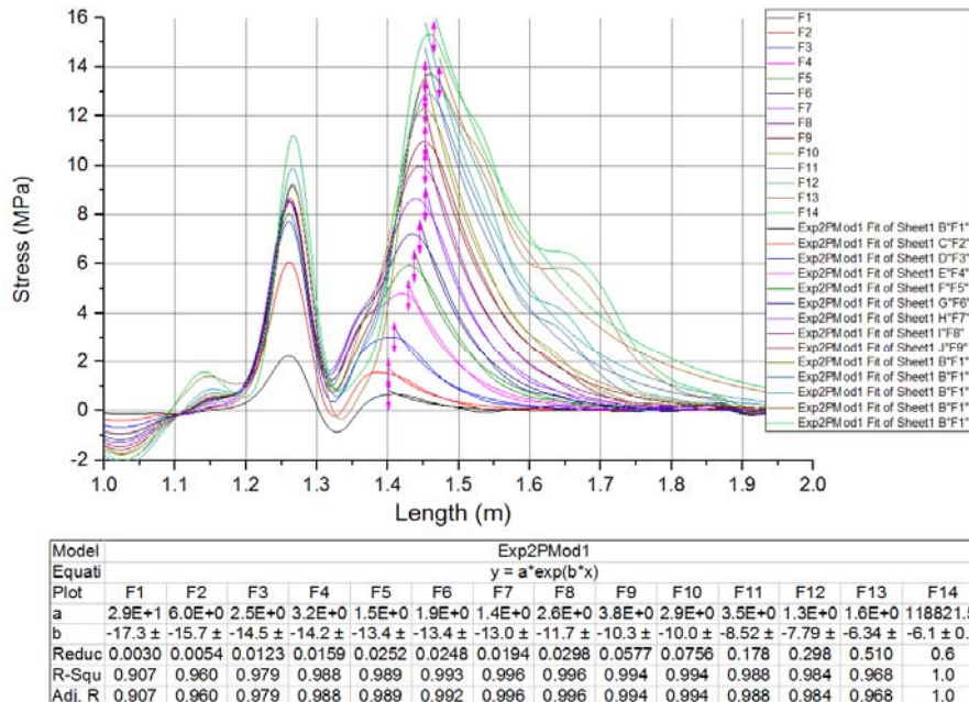
Figure 200 Détermination du coefficient \alpha à partir des contraintes de cisaillement dans les parties barre-scellement collées
