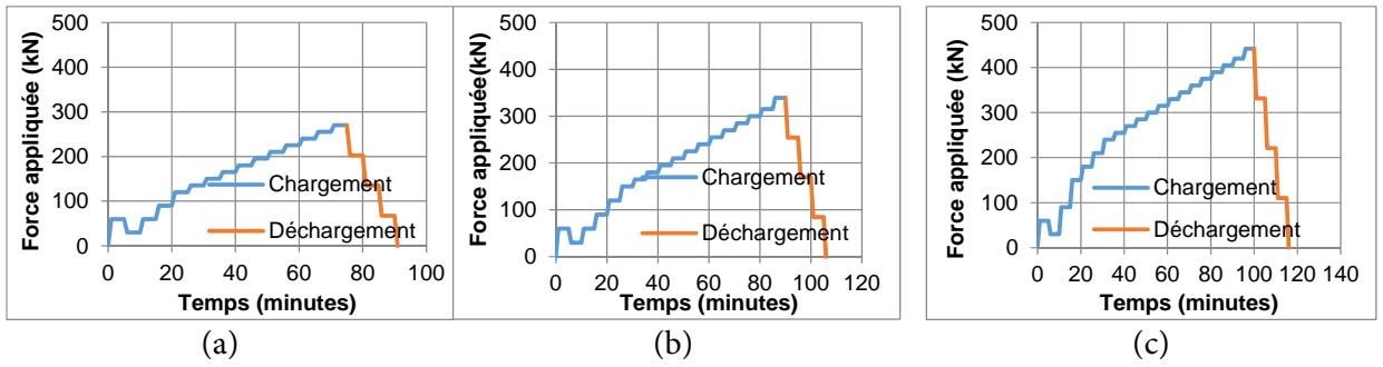
Figure 181 Programmes de chargement/déchargement pour les 3 diamètres de barre : a) 25mm ; b) 28mm ; c) 32mm.
