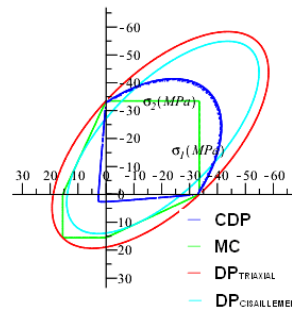
(f) Surfaces de plasticité en état plan de contraintes
