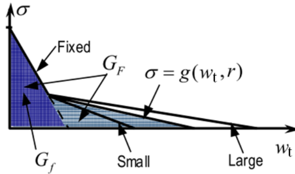
Figure 71 Modèle de fissure cohésive (d'après Bazant & Yu, 2004)
