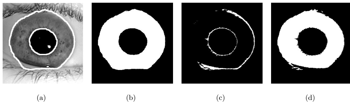
FIGURE 5.6 – Masque de l’iris résultant du module de segmentation d’OSIRIS-V4. Affichage des contours précis sur l’image Originale (a). Masque de la région de l’iris par les contours précis (b). Masque des autres occlusions par le seuillage adaptatif (c). Masque final de l’iris (d).
