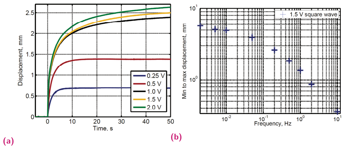
Fig. C.19. (a) Réponse d'actionneurs PEDOT: PSS / PVDF greffé PEGMA / PEDOT: PSS pour différentes tensions d'actionnement et (b) Amplitude de déplacement de ces mêmes actionneurs pour différentes fréquences.
