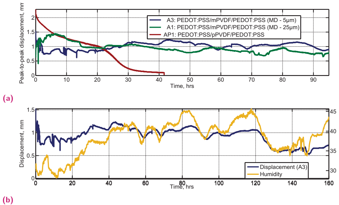
Fig. C.20. (a) Mesure de la durée de vie d'actionneurs hybrides PVDF greffé PEGMA (mPVDF) et de membranes vierges (PVDF). La profondeur d'interaction entre le PEDOT: PSS et la mPVDF est indiquée dans la légende. (b) Amplitude du déplacement d'un actionneur PEDOT: PSS / PVDF-greffage PEG / PEDOT: PSS avec un MD de 5 \mu m dans un liquide ionique (bleu) et changement de l'humidité de l'environnement (jaune)
