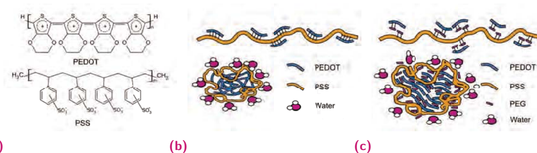
Fig. C.3. (a) Structure chimique du PEDOT :PSS et illustration schématique de la structure cœur/coquille dans une solution aqueuse (b) sans et (c) avec des additifs secondaires.
