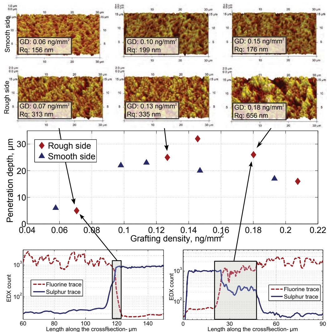
Fig. C.12. (Bas) Spectres EDX pour le soufre (bleu trait plein) et le fluor (rouge ligne pointillée) le long des sections transversales du PEDOT: PSS / PVDF avec greffage PEGMA. La densité de greffage (GD) est indiquée par les flèches. (Centre) Profondeurs de greffage par rapport à la densité de greffage (GD) tracées séparément pour du PEDOT: PSS déposé sur le côté rugueux ( \Delta bleu) et le côté lisse ( \diamond rouge) de la membrane PVDF avec greffage PEGMA. (Haut) Images obtenues par microscopie à force atomique (AFM) des surfaces lisses et rugueuses de membranes PVDF avec greffage PEGMA pour différentes densités de greffage (GD). La densité de greffage et la rugosité sont indiquées dans les légendes.
