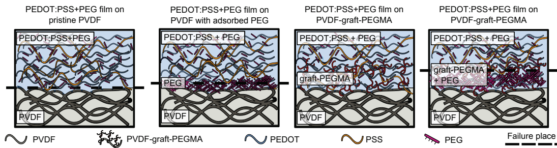
Fig. C.16. Représentation schématique de différentes méthodes de fonctionnalisation du PVDF et leur influence sur l'adhésion avec du PEDOT :PSS.
