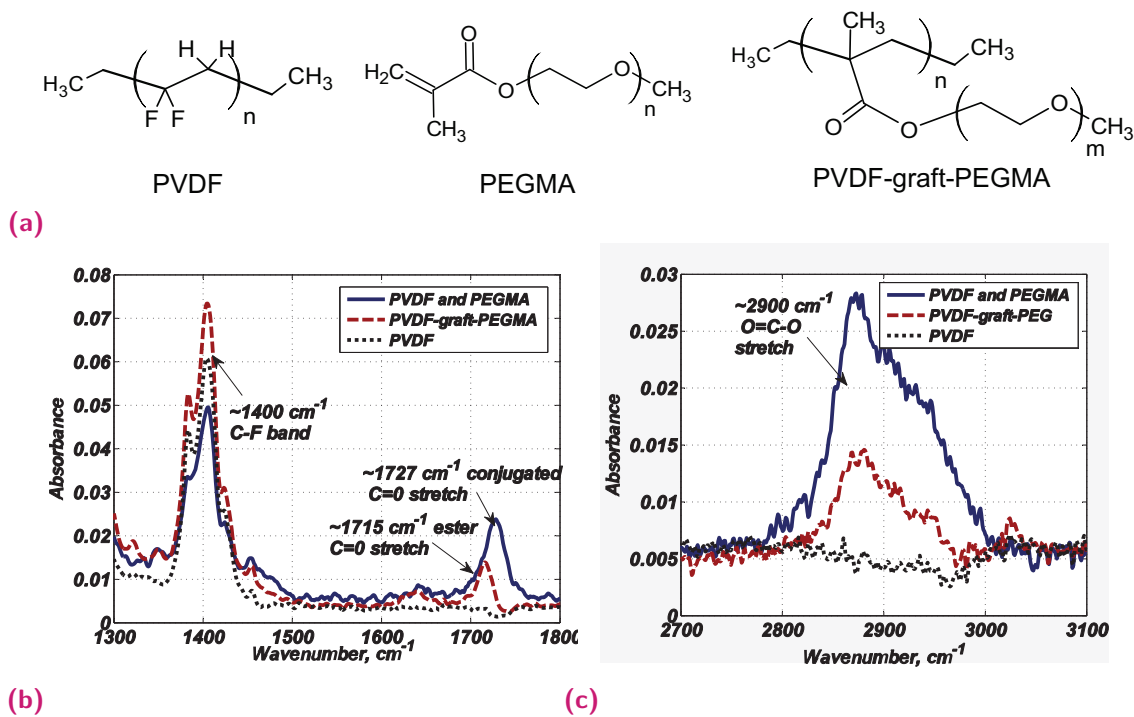
Fig. C.8. (a) Structure chimique du PVDF, du PEGMA et du PVDF-PEGMA et leur signature entre (b) 1300 – 1800 cm -1 et (c) 2700 – 3100 cm -1
