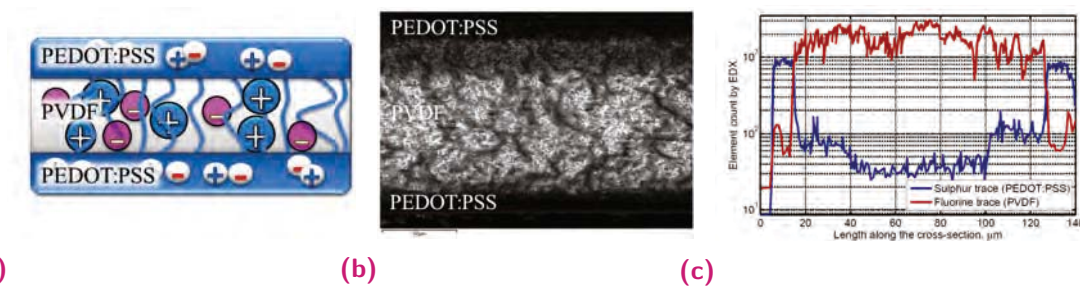
Fig. C.6. (a) Représentation schématique d'un actionneur PEDOT: PSS / PVDF / PEDOT: PSS avec des électrodes percolées (lignes bleues). (b) Image SEM d'une coupe transversale de l'actionneur tricouche avec du PEDOT: PSS dans la membrane PVDF (c) Spectres EDX le long de la coupe transversale faisant apparaître clairement des traces de soufre (PEDOT: PSS) en bleu et de fluor (PVDF) en rouge. Les traces de soufre significativement plus élevées que zéro traduisent un phénomène de percolation dans la membrane.
