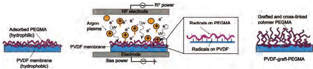
Fig. C.7. Illustration schématique d'un greffage lors de l'irradiation plasma : (1) Immobilisation du monomère ou macromonomère à la surface du substrat; (2) activation des deux: la surface du polymère et le précurseur du monomère par plasma en créant des radicaux sur chacun; (3) Réaction simultanée entre les espèces actives conduisant à la réticulation du polymère et du substrat. Si on utilise du PEGMA comme précurseur de la réaction et le PVDF en tant que substrat, cette procédure conduit à une hydrophilisation de la surface du PVDF en surface.
