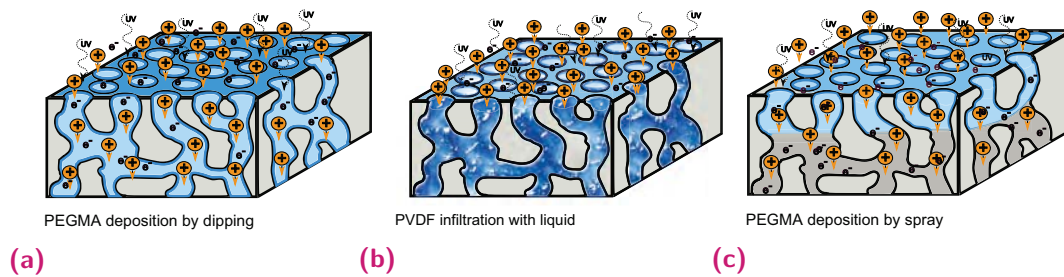
Fig. C.9. Schémas illustrant trois stratégies différentes de dépôt de précurseur et l'interaction du plasma à la surface de la membrane: (a) dle dépôt par trempage dans une solution diluée contenant le précurseur et conduisant à son adsorption sur la surface de la membrane suivi de l'activation du greffage par plasma sur toute l'épaisseur; (b) le dépôt par immersion dans un liquide visqueux qui empêche la pénétration du plasma et l'activation des pores; (c) le dépôt par pulvérisation qui limite le dépôt du précurseur à une certaine profondeur.
