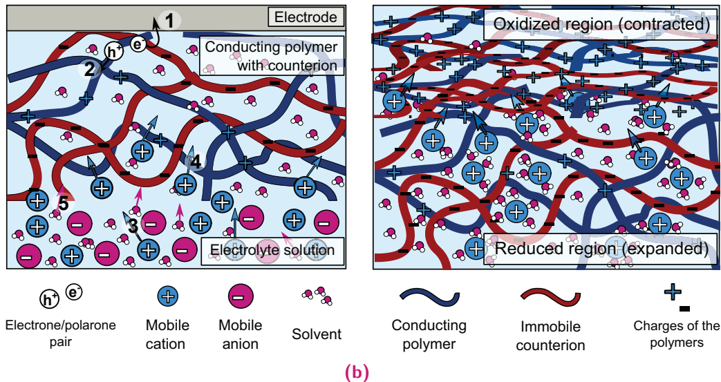
Fig. C.2. (a) Illustrations schématique du processus qui entre en jeu lors de la dilatation volumique ① les électrons sont supprimés de la chaîne polymère ② les polarons créés se propagent le long des chaînes polymères et engendrent un changement de conformation du polymère ③-④ les cations se déplacent vers l'électrolyte à travers l'interface et entre les chaînes polymères et ainsi ouvrent des canaux au sein du polymère ⑤ si elles sont présentes, les molécules du solvant peuvent pénétrer le film polymère. (b) Structure du polymère dans son état oxydé et réduit. A cause de la charge nette induite par le changement de conformation du polymère et due à la présence des ions et du solvant, l'état réduit est plus ouvert. D'un autre côté, l'état oxydé est plus compact et contient moins de molécules d'eau et réduit fortement la mobilité des ions.
