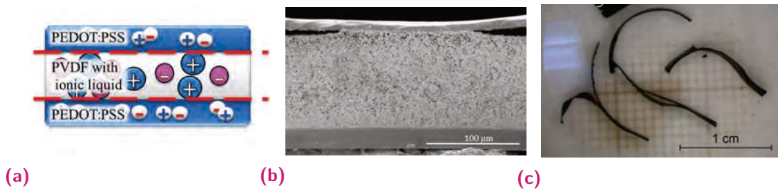
Fig. C.5. (a) Illustration schématique d'actionneurs PEDOT: PSS / PVDF / PEDOT: PSS avec un liquide ionique avec une défaillance potentielle dans la zone d'adhésion entre les couches (ligne pointillée rouge). (b) Image par microscopie à balayage (MEB) d'une coupe transversale de l'actionneur tricouche où l'on peut observer très clairement la délamination de la couche de PEDOT: PSS de la membrane PVDF (c) Actionneurs avec une mauvaise adhésion interfaciale après immersion dans un liquide ionique.
