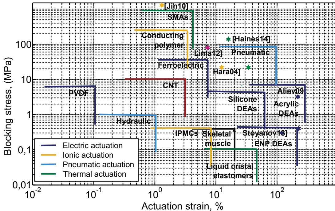
Fig. C.1. Contrainte en fonction de la déformation pour différents types de muscles artificiels et d'actionneurs. Types d'actionnement : bleu-électrique, orange-ionique, vert-thermique, rouge-nanotubes de carbone, gris-autres, noir-muscles naturels de mammifères. Adapté de [249, 269] et d'autres références citées dans le texte.
