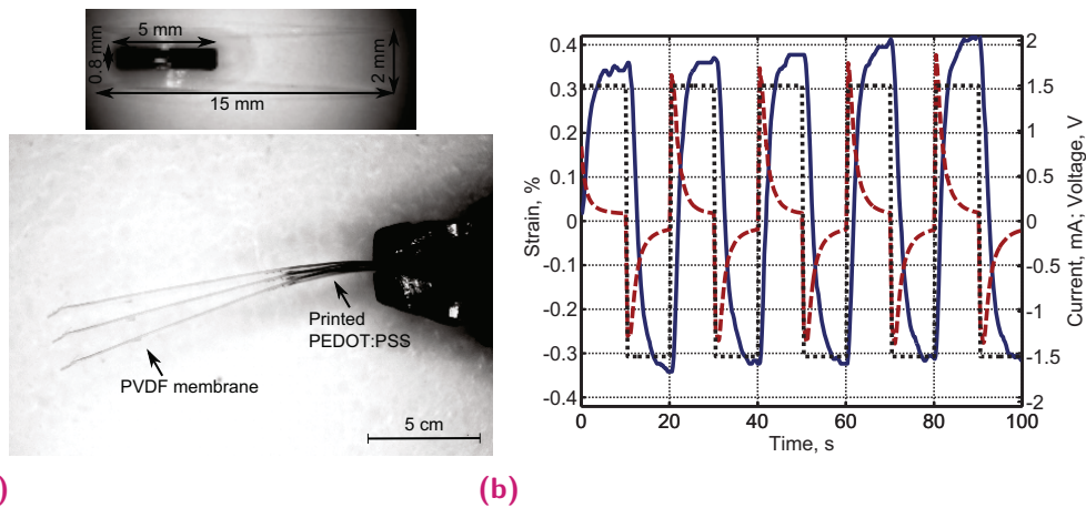
Fig. C.22. (a) Images fusionnées de l'actionneur dans sa position initiale et de ses extrémités lors de l'actionnement avec un signal carré de 1.5 V à 50 mHz . La position de la couche de PEDOT :PSS imprimée est indiquée par des flèches. Les dimensions de l'actionneur utilisé (2x15 mm ) et couche de PEDOT: PSS imprimée (0.8x5 mm ) sont indiqués ci-dessus. (b) Déplacement (ligne bleue) et courant transféré (ligne pointillée rouge) pour des actionneurs imprimés (10 couches, 0.36 mg ) lors de l'actionnement. La forme du signal de tension utilisé est indiquée en pointillé noir.
