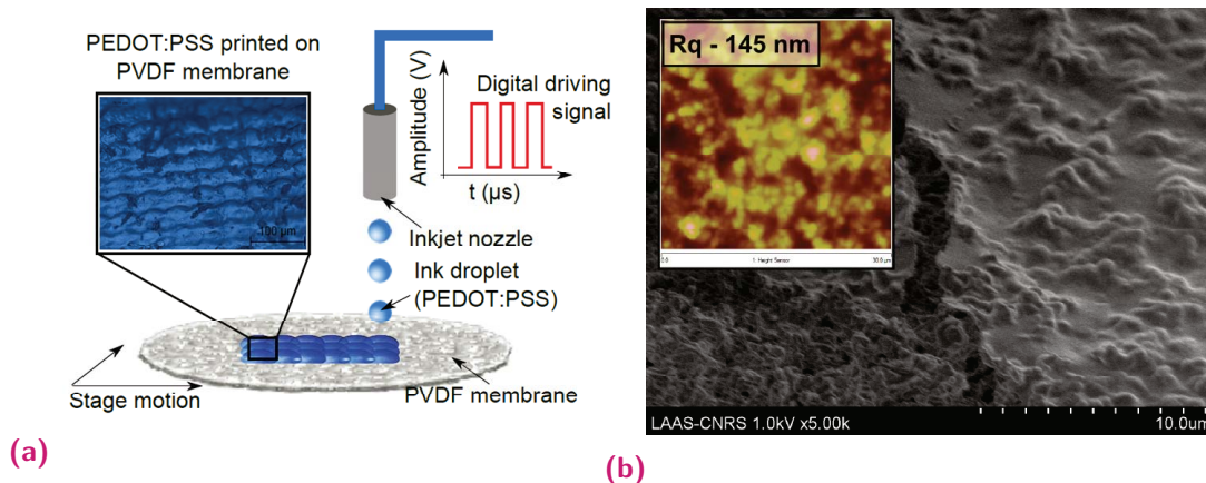
Fig. C.21. Illustration schématique d'une impression jet d'encre piézo-électrique: une tension électrique est utilisée pour déformer le matériau piézo-électrique et générer une impulsion de pression dans le fluide, qui éjecte ensuite une gouttelette d'encre (PEDOT: PSS) à partir de la buse; un motif est généré par le déplacement de la tête d'impression par rapport au substrat (membrane de PVDF) en deux dimensions. En médaillon : Photo prise avec un microscope optique après l'impression de 20 couches de PEDOT: PSS.
