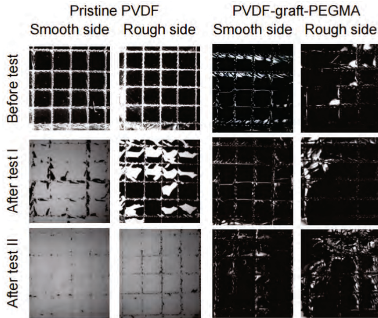
Fig. C.15. Test d'adhésion du PVDF et de membranes PVDF avec un greffage PEGMA (blanc) et PEDOT: PSS (noir). Les photos sont prises après que la grille a été découpée (avant le test), après 5 tests consécutifs de décollement (test I) et de nouveau après une incubation de la bicouche dans le liquide ionique pour 24 heures et 5 tests supplémentaires de décollement (test II).
