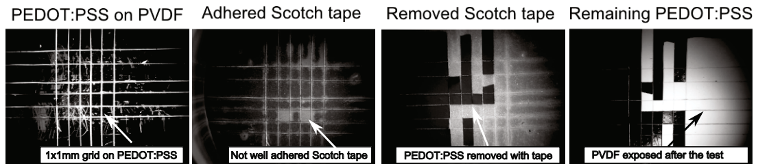
Fig. C.14. Étapes du processus d'évaluation d'adhésion (de gauche à droite): grille de 25 cases découpées sur le PEDOT: PSS jusqu'à la membrane de PVDF; Un ruban adhésif de type Scotch™ est appliqué sur la grille pour effectuer le test d'adhésion ; image du ruban adhésif après qu'il a été retiré du film; image de la membrane PVDF et du PEDOT :PSS restant sur la membrane après que le ruban adhésif a été retiré
