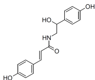
p -coumaroyl-octopamine
