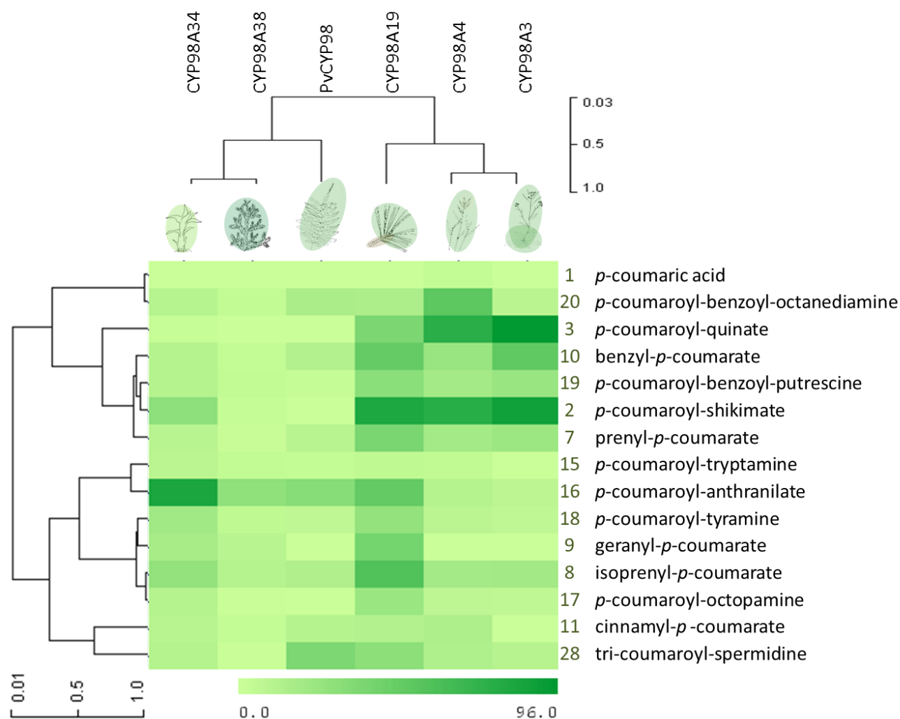
Figure 5.4 Classification hiérarchique des substrats et P450s testés biochimiquement.
