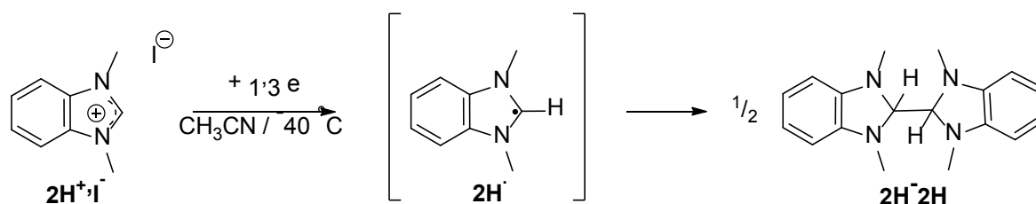
Schéma III-4. Synthèse de 2H-2H
