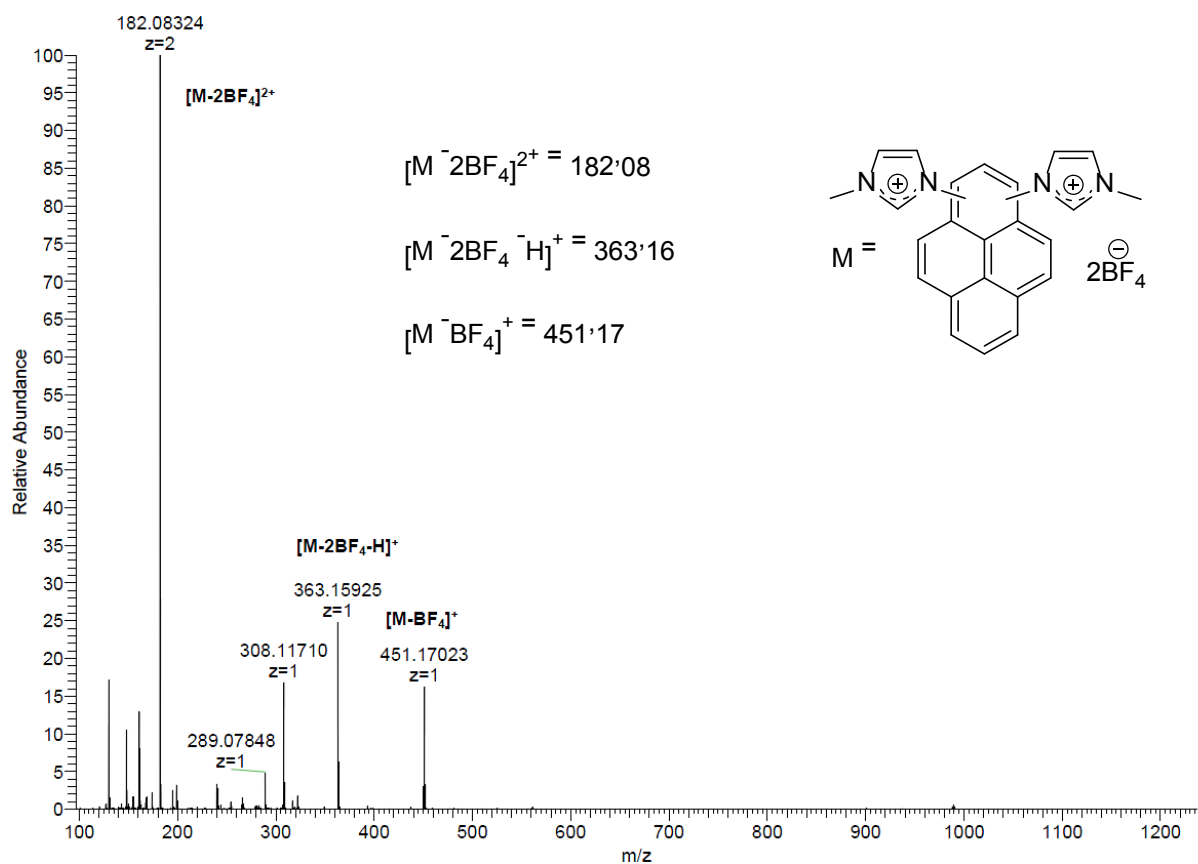
Figure IV-8. Spectre de masse ESI du brut réactionnel après oxydation de 13H^+, BF_4^- en présence de 1-méthylimidazole
