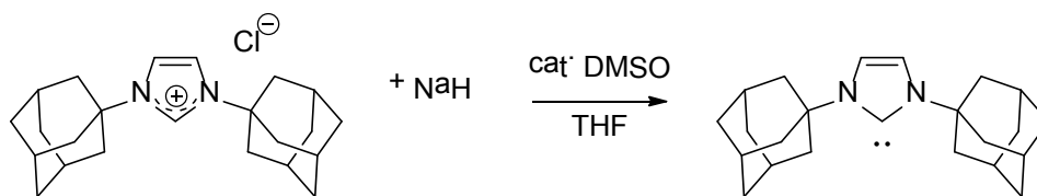
Schéma I-2. Préparation du premier NHC libre isolé par Arduengo 3
