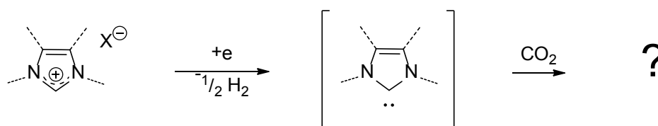
Schéma I-11. Principe proposé
