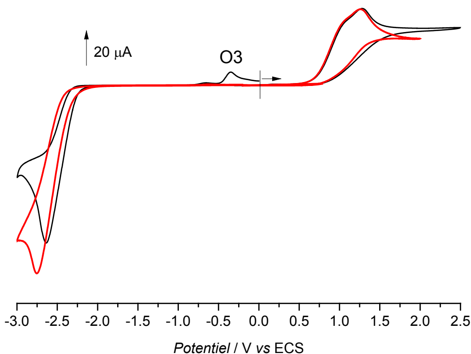
Figure I-14. Voltammogrammes cycliques de 5\mathbf{H}^+, \mathbf{HC}_2\mathbf{O}_4^- sous argon (en noir), et sous \text{CO}_2 (en rouge) ( \text{CH}_3\text{CN} , C = 3,1 \times 10^{-2} \text{ M} , 0,1 \text{ M TBAPF}_6 ; électrode de travail : carbone; électrode de référence : ECS ; contre-électrode : platine ; \varnothing = 1 \text{ mm} , \nu = 0,1 \text{ V s}^{-1} ; température ambiante)
