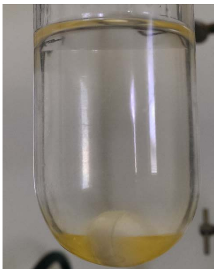
Image II-1. Séparation de phase entre 5\text{H}^+, \text{HSO}_4^- et le myristate d'isopropyle
