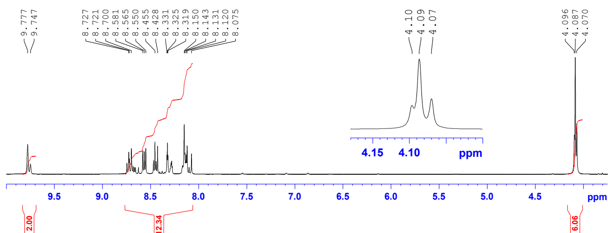
Figure IV-9. Spectre RMN ^1H de 14H^{2+}, 2BF_4^- à 16H^{2+}, 2BF_4^- (DMSO- d_6 , 300 MHz, 298 K)
