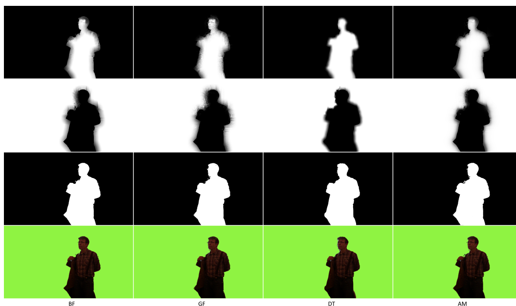
FIGURE 3.23 – Comparaison de l’utilisation des différents filtres pour la méthode d’affinage de la silhouette. Les deux premières lignes illustrent les cartes de diffusion du premier plan et de l’arrière plan. La troisième ligne illustre la silhouette obtenue. Enfin, la dernière ligne affiche le compositing avec l’image couleur. Dans l’ordre des colonnes : Filtre bilatéral joint (BF), Filtre guidé (GF), Filtre domain transform (DT), Filtre adaptive manifold (AM).
