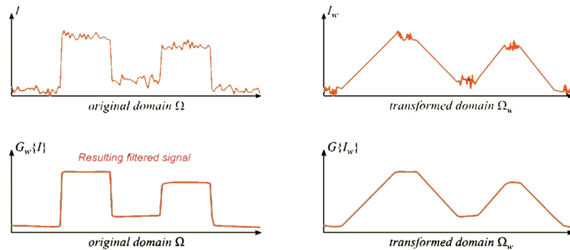
FIGURE 3.19 – Principe du filtre domain transform sur un signal en 1 dimension. Le signal est transformé dans un domaine \Omega_w et filtré spatialement dans ce domaine. Le signal filtré est ensuite reporté dans le domaine original. Cette opération filtre le signal en conservant les variations importantes. Elle est efficace en terme de complexité et coût mémoire.
