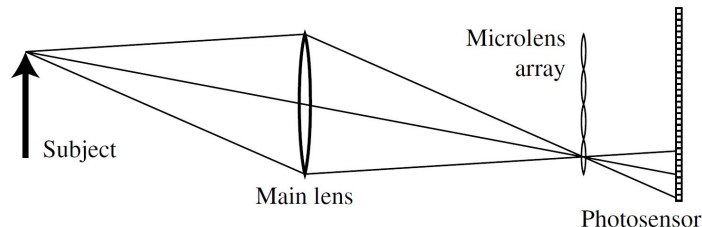
FIGURE A.3 – Principe du capteur plénoptique. Un réseau de micro-lentille est inséré entre l’optique et le capteur. Image tirée de [NLB + 05].
