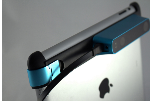
FIGURE 2.7 – Capteur Occipital de la société Structure basé sur la technologie de lumière structurée de la société Primesense . Le capteur est ici monté sur un appareil mobile iPad .
