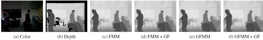
FIGURE C.11 – Les trous d'une image de profondeur issue d'une Kinect sont obstrués avec une méthode d' inpainting FMM puis GFMM. Un filtrage guidé est effectué pour atténuer le bruit et affiner les contours. (Illustration tirée de [LGL12])
