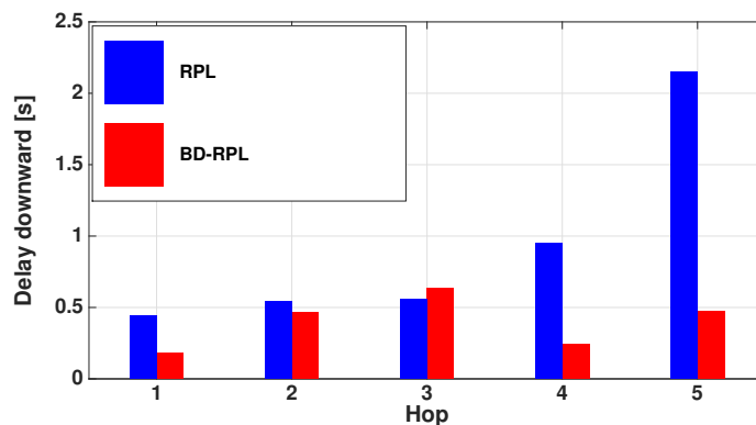
FIGURE 5.8 – Délai de transmission descendant en fonction de la distance en nombre de sauts.
