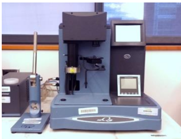
Figure 2.19 Thermogravimetric analysis (TGA) instrument (Laboratoire Procédés et Ingénierie en Mécanique et Matériaux, PIMM, ENSAM, Conservatoire National des Arts et Métiers, CNAM, Paris).
