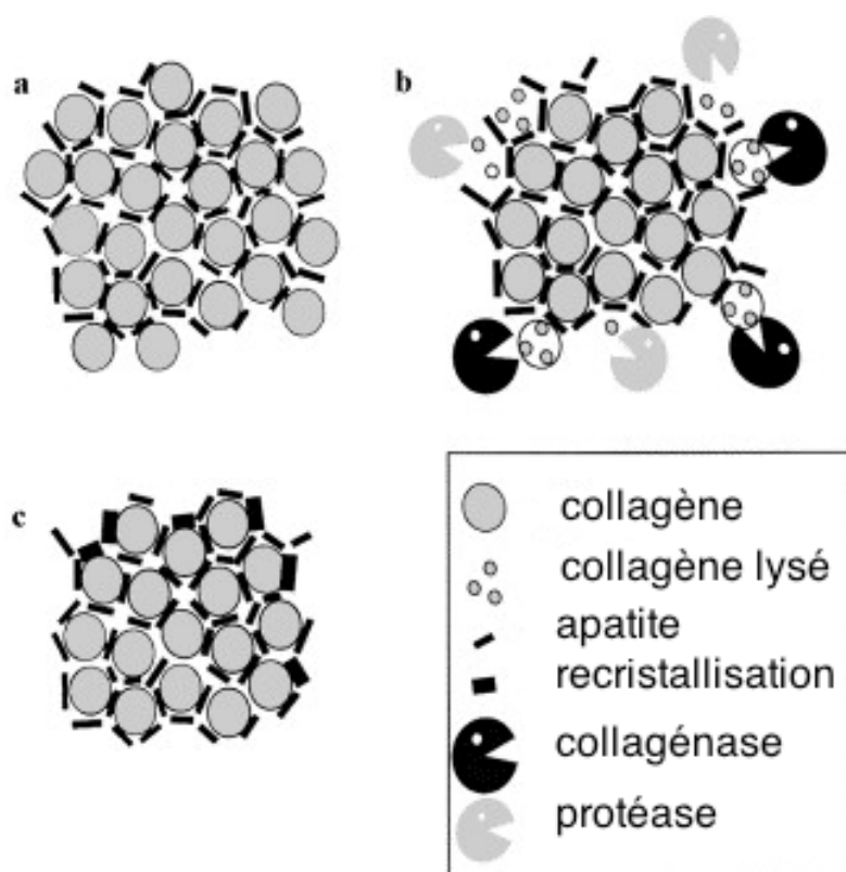
Figure 25 : Théorie de l'exclusion enzymatique (adapté de Nielsen-Marsh et al. , 2000)
