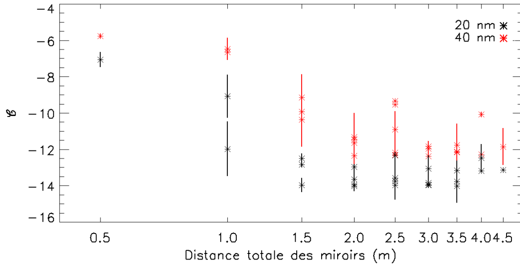
FIGURE 2.31 – Contraste en échelle logarithmique (astérisques) en fonction de la distance totale entre les miroirs déformables pour une quantité d’aberrations totale sur le montage optique de 20 nm (en noir) et de 40 nm (en rouge). Les lignes correspondent à la dispersion des valeurs de contraste.
