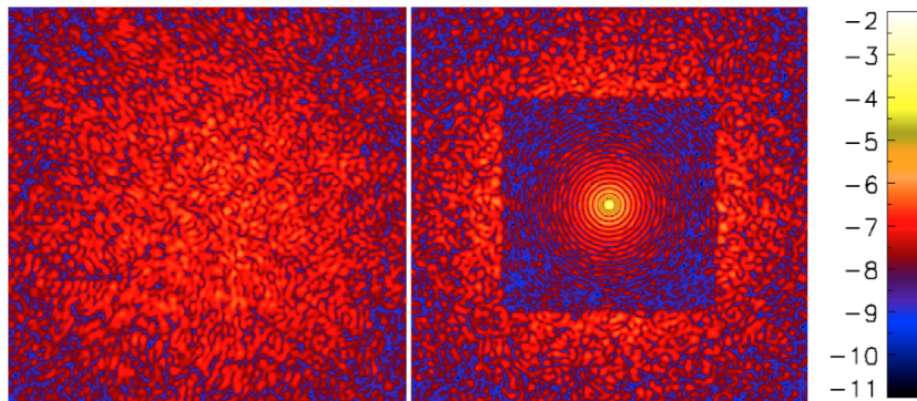
FIGURE 1.11 – FÉP en échelle logarithmique avec turbulence atmosphérique (modèle de Kolmogorov et paramètre de Fried de 0.2) avant (à gauche) et après (à droite) correction d'un miroir déformable constitué de 2 000 actionneurs.
