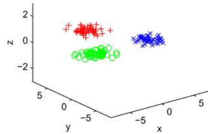
Projection des données suivant la distance pondérée après apprentissage de la métrique
