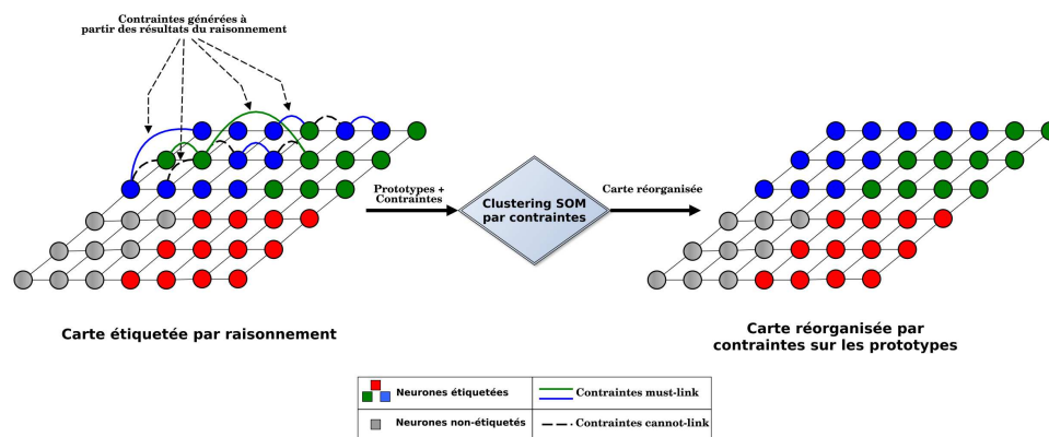
FIGURE 8.2 – Vue générale d'une prise en compte des résultats du raisonnement pour la réorganisation des résultats de SOM
