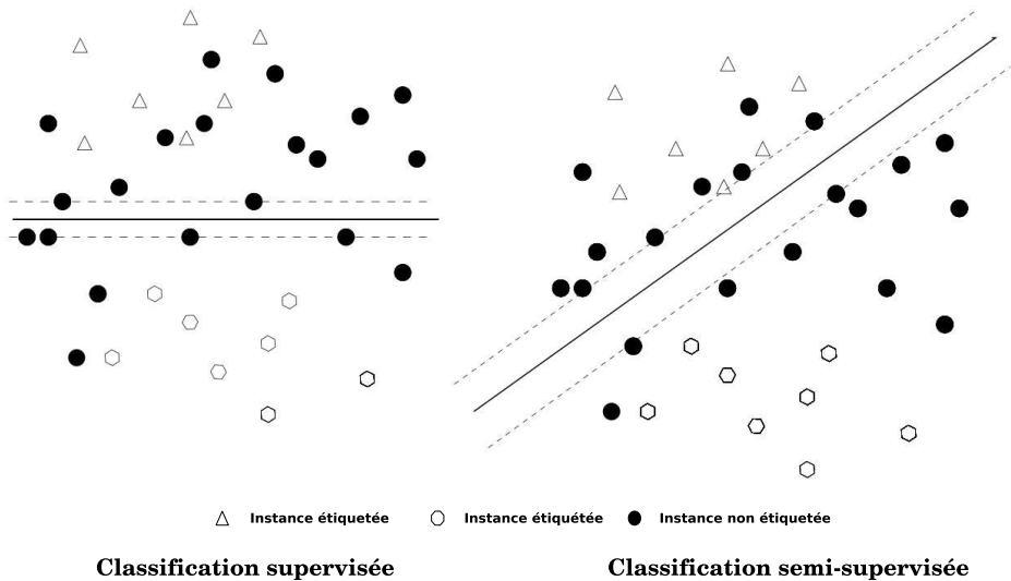
FIGURE 5.7 – Illustration de l'apport des données étiquetées pour la classification, figure inspirée de BENNETT et DEMIRIZ (1999)
