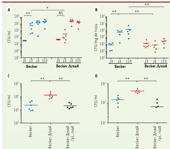
Figure 2. Impact de RsaA sur la virulence in vivo chez la souris. Deux modèles d'infection in vivo ont été développés : un modèle d'infection sur cathéter (pour mimer une infection chronique) et un modèle de bactériémie (pour mimer une infection aiguë). La quantification des bactéries vivantes dans le cathéter (A) et dans les tissus environnants (B) 3, 6 et 10 jours post-infection a été réalisée par numération sur boîtes gélosées. Les résultats sont exprimés en nombre de CFU/ml (A) ou par mg de tissu (B). Chaque point désigne le nombre de bactéries par souris et la ligne noire représente la moyenne pour chaque condition testée. Le second modèle a été réalisé par injection intrapéritonéale de 1 \times 10^8 bactéries. Après 3 h d'infection, les bactéries viables dans la cavité péritonéale (C) ou dans le sang (D) ont été dénombrées. Les résultats sont exprimés en nombre de CFU/ml. Les différences statistiques * ( p < 0,05 ) et ** ( p < 0,005 ) entre 2 groupes ont été obtenues par un test de Mann-Whitney. NS : non significatif.
