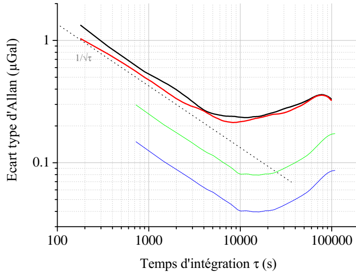
FIG. 3.14 – Ecart type d'Allan d'une mesure de g de 5 jours faite alternativement en compensant l'asymétrie de notre interféromètre (ligne rouge) et sans la compenser (ligne noire). La ligne bleue représente l'écart-type d'Allan du biais sur g calculé à partir de la mesure des fluctuations de la vitesse initiale des atomes au cours des 5 jours de mesure pour un interféromètre utilisant une fréquence de Rabi de 12,5 \text{ kHz} \times 2\pi . La ligne verte est l'écart-type d'Allan qu'on aurait obtenu si nous avions utilisé une fréquence de Rabi deux fois plus importante pour cette mesure.
