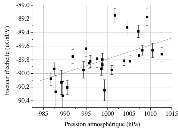
FIG. 4.15 – Corrélation entre les variations du facteur d'échelle et les variations de la pression atmosphérique.
