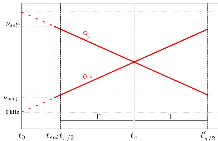
FIG. 2.15 – Rampes appliquées sur la fréquence des impulsions Raman pour les deux configurations k_\uparrow et k_\downarrow . Un saut sur la fréquence initiale de la configuration \uparrow est appliqué pour que les fréquences des trois impulsions de l'interféromètre délivrées par la DDS soient symétriques par rapport à l'impulsion \pi .
