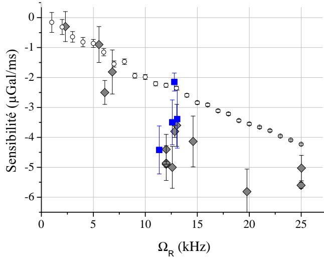
FIG. 3.6 – Sensibilité de la mesure de g aux variations de la date de lâcher des atomes selon la fréquence de Rabi. Les losanges gris sont le résultat de mesures et les ronds blancs de simulation. Les carrés bleus représentent la mesure de cette sensibilité déterminée en faisant varier la classe de vitesse sélectionnée.
