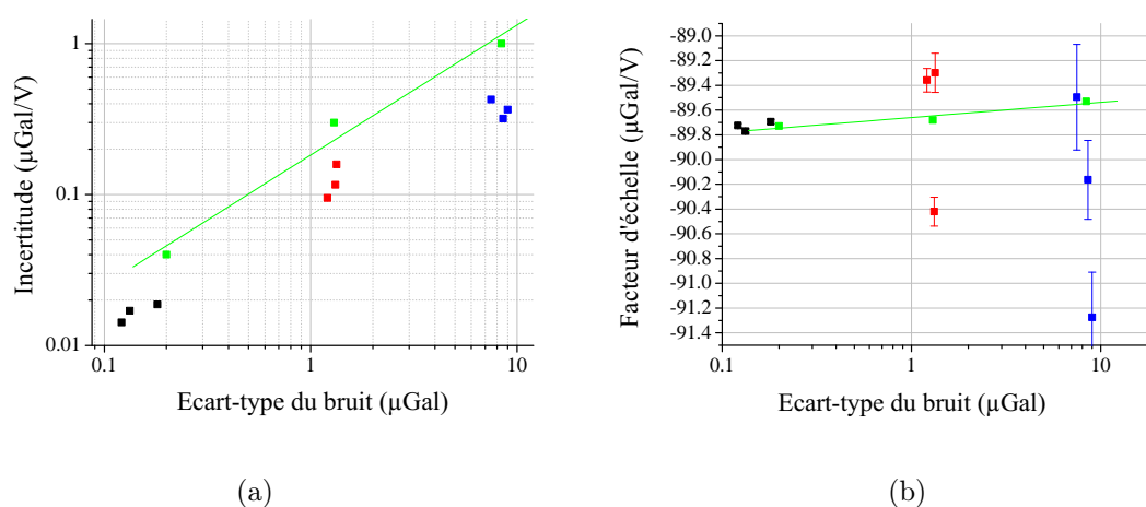
FIG. 4.12 – Variations de l'incertitude (a) et du facteur d'échelle (b) selon l'écart-type du bruit résiduel, lorsque le facteur d'échelle est déterminé par le CAG (en rouge), par le FG5 (en bleu), le signal synthétique de g (en bleu) et le résultat de simulation de l'étalonnage (en vert).
