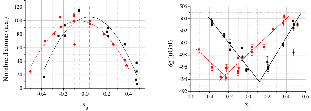
FIG. 2.11 – Effet de la variation des rapports d'intensité dans le MOT-3D. Graphique de gauche: mesure du nombre d'atomes selon le rapport des puissances du MOT x_{12} (en noir) et du rapport x_{34} (en rouge). Graphique de droite: variations de g selon les rapports d'intensités x_{12} et x_{34} .
