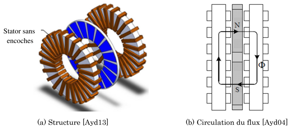
Figure 1.30 : AFIR à stator non encoché et bobinage toroïdal
