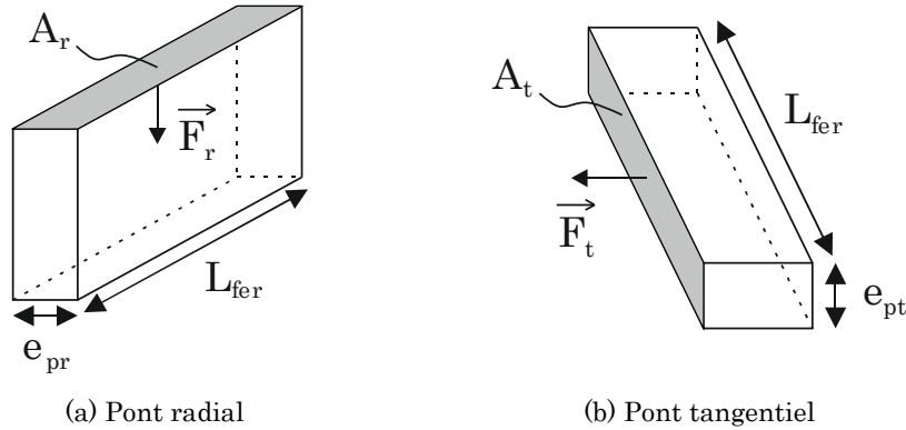
Figure 3.62 : Dimensions géométriques des ponts radial et tangentiel
