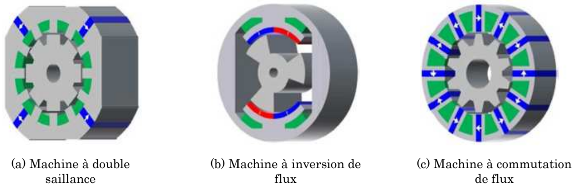
Figure 1.12 : Machines synchrones à aimants permanents au stator [Zhu14]
