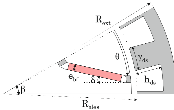
Figure 4.3 : Variables géométriques de l'optimisation
