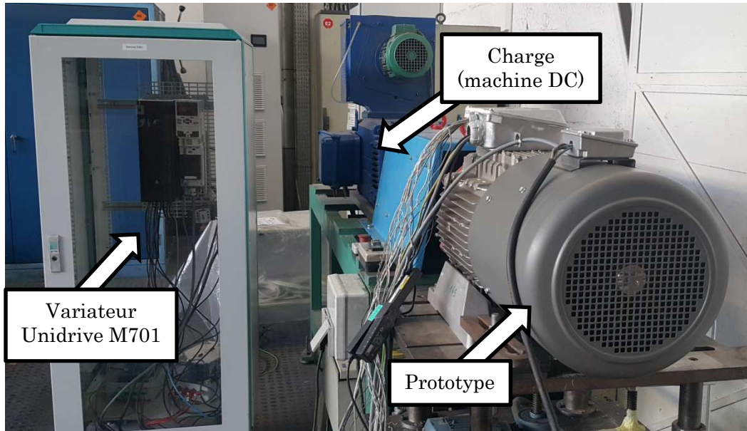
Figure 4.14 : Banc expérimental
