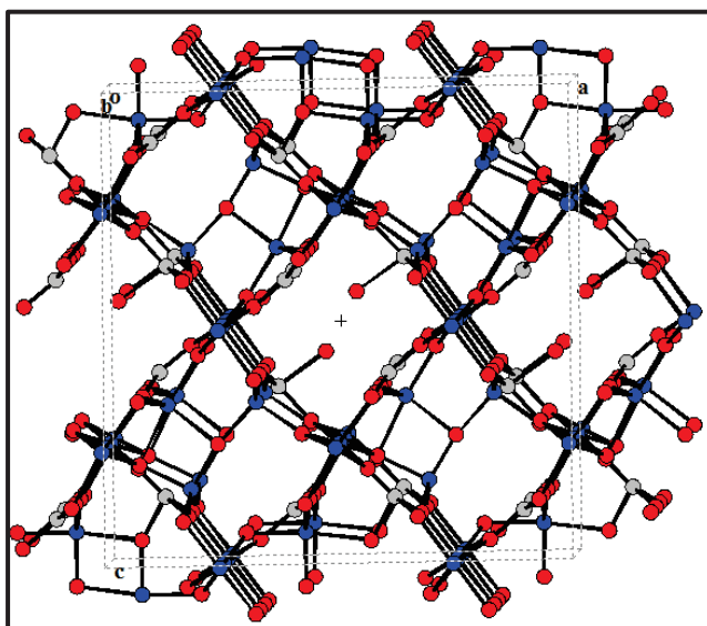
Figure 14 : Représentation de la structure \text{Al}_4\text{B}_2\text{O}_9 projetée dans le plan (ac).
