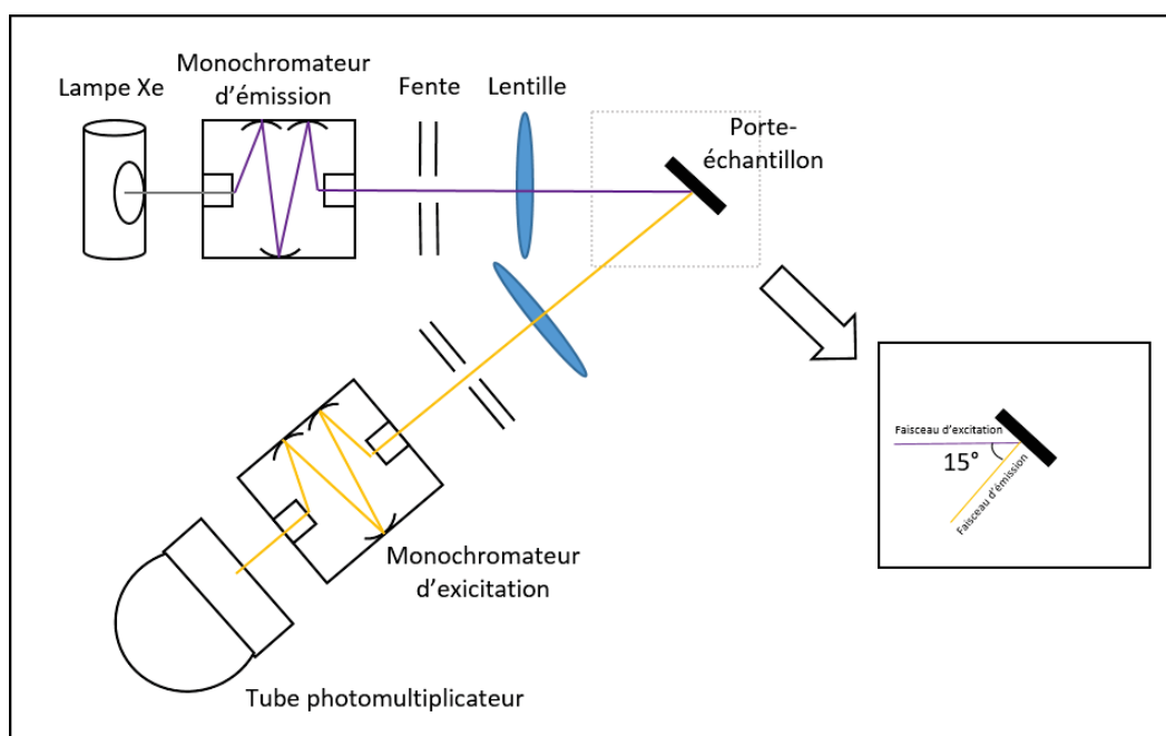
Figure 3 : Schéma du spectromètre Fluorolog, appelé spectrophotomètre n°3.
