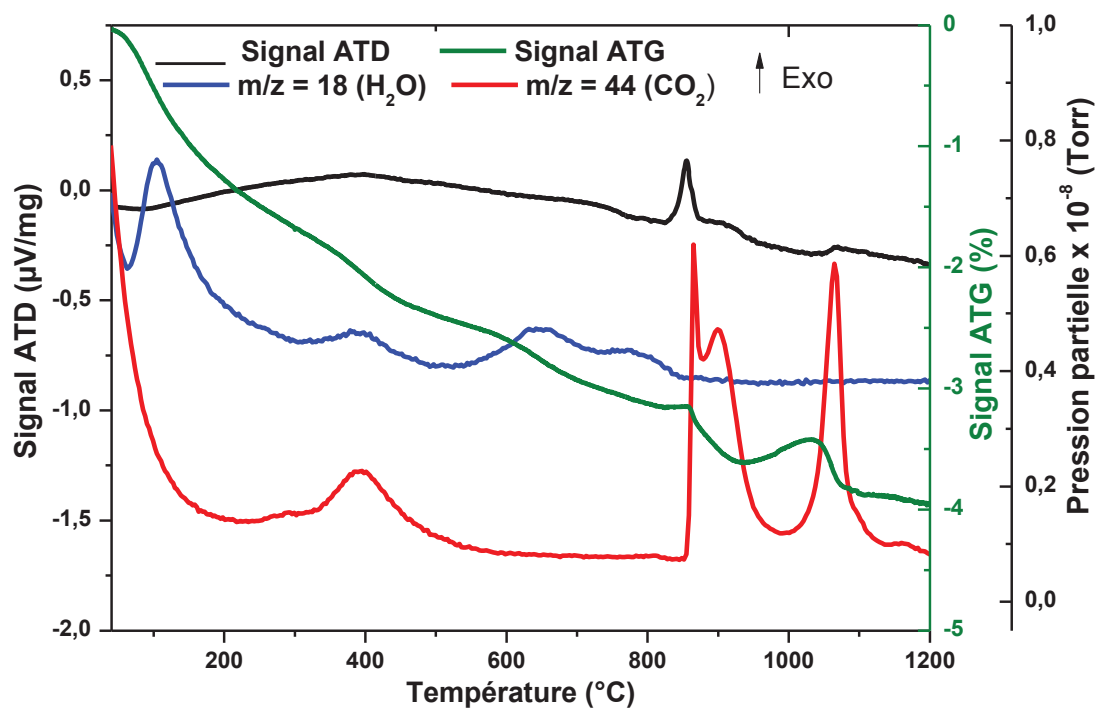
Figure 7 : Courbes d'ATD-TG-SM d'une poudre de YAB SG-n de granulométrie centrée autour de 6 µm recuite au préalable sous O 2 à 550°C, sous O 2 avec une vitesse de chauffe de 5°C/min.
