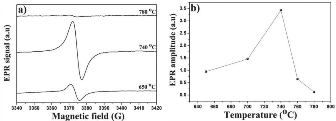
Figure 19 : a) Spectres RPE bande X des poudres de YAB PP calcinées à 650 °C, 740°C et 780°C, b) Intensité du signal RPE de poudres de YAB PP calcinées entre 650°C et 780°C à (g = 2,002) en fonction de la température de calcination, issu de [111].
