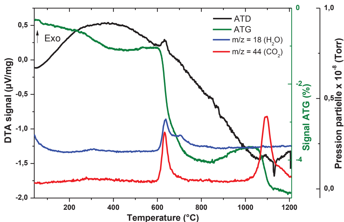
Figure 6 : Courbes d'ATD-TG-SM d'une poudre de YAB SG-n de granulométrie centrée autour de 60 µm recuite au préalable sous O 2 à 550°C, analysée sous O 2 avec une vitesse de chauffe de 5°C/min.
