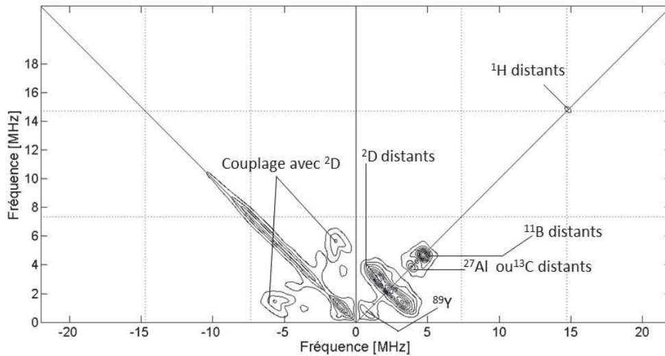
Figure 33 : Spectre RPE HYSORE bande X ( \tau = 136 ns) acquis à 75 K d'une poudre de YAB SG-n synthétisée avec de l'acide propionique deutéré calcinée à 450°C. Spectre normalisé à 1, courbes de niveau tracées pour les valeurs suivantes 0,1 ; 0,2 ; 0,3 ; 0,4 ; 0,5 ; 0,6 ; 0,7 ; 0,8 ; 0,9. Les lignes pointillées représentent les points aveugles.
