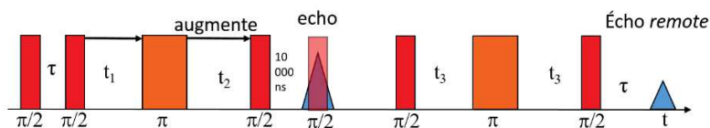
Figure 7 : Schéma de la génération d'un écho stimulé lors d'une séquence RPE à 7 impulsions, appelée HYSORE remote .
