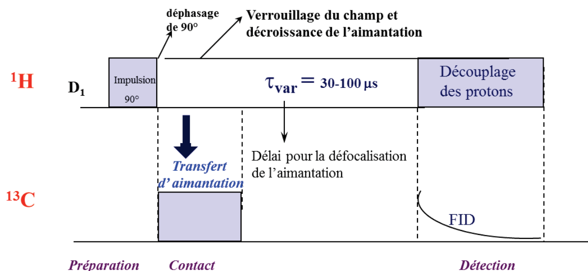
Figure 6 : Schéma d'une séquence de RMN 13 C DD.
