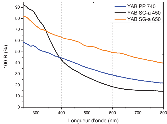
Figure 7 : Spectres de réflectance diffuse des poudres de YAB PP pyrolysées à 700°C puis calciné à 740°C (courbe bleue), YAB SG-a calcinée à 450°C (courbe noire) et à 650°C (courbe orange).
