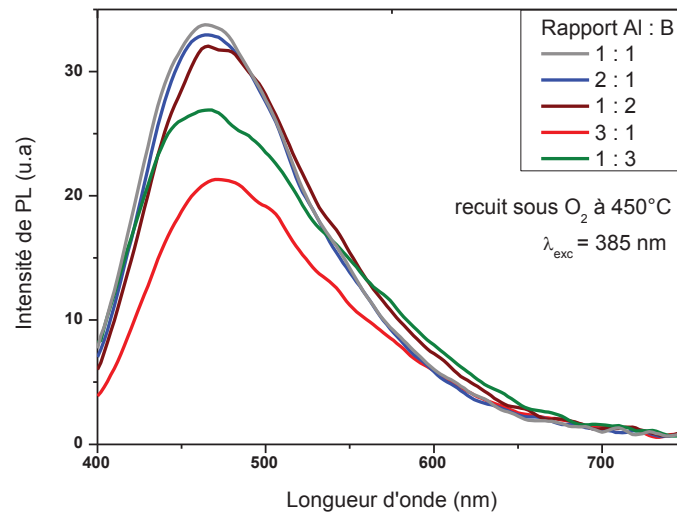
Figure 26 : Spectres d'émission de poudres d'aluminoborates en fonction de la composition, excités à 385 nm. Spectres mesurés avec le spectrophotomètre n°1 (annexe 5).
