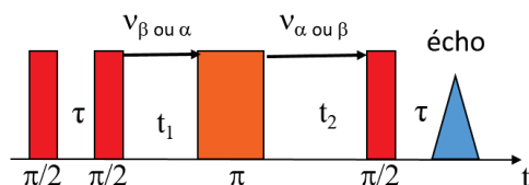
Figure 6 : Schéma de la génération d'un écho stimulé lors d'une séquence RPE à 4 impulsions, appelée HYSORE.
