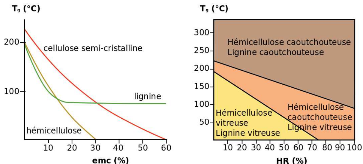
FIGURE 1.20 – Température de transition vitreuse ( T_g °C) : pour chaque composant polymérique du bois, en fonction de l'humidité interne (emc %) (gauche); pour la matrice hémicellulose - lignine, en fonction de l'humidité relative (HR %) (droite), d'après (Salmén 1982) et (Salmén 1986), lu dans (Navi 2011).
