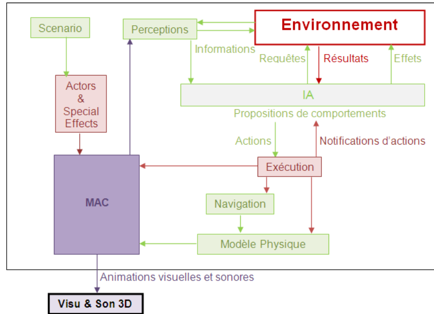
FIGURE 4.5 – Organisation générale des modules du projet Terra Dynamica
