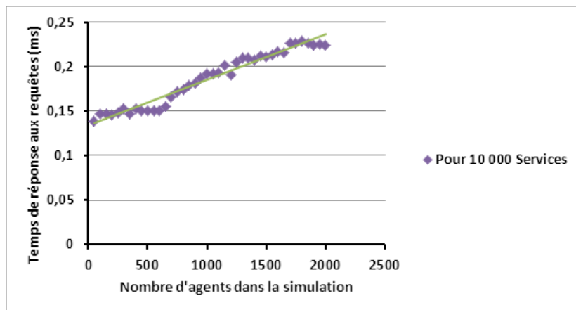
FIGURE 4.11 – Temps de réponse moyen pour 10 000 services et 2 500 agents
