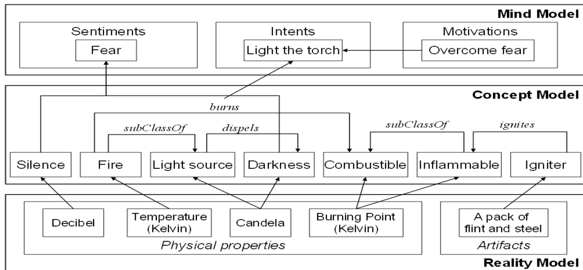
FIGURE 2.8 – Architecture du framework à trois couches proposé dans [Chang et al., 2005]
