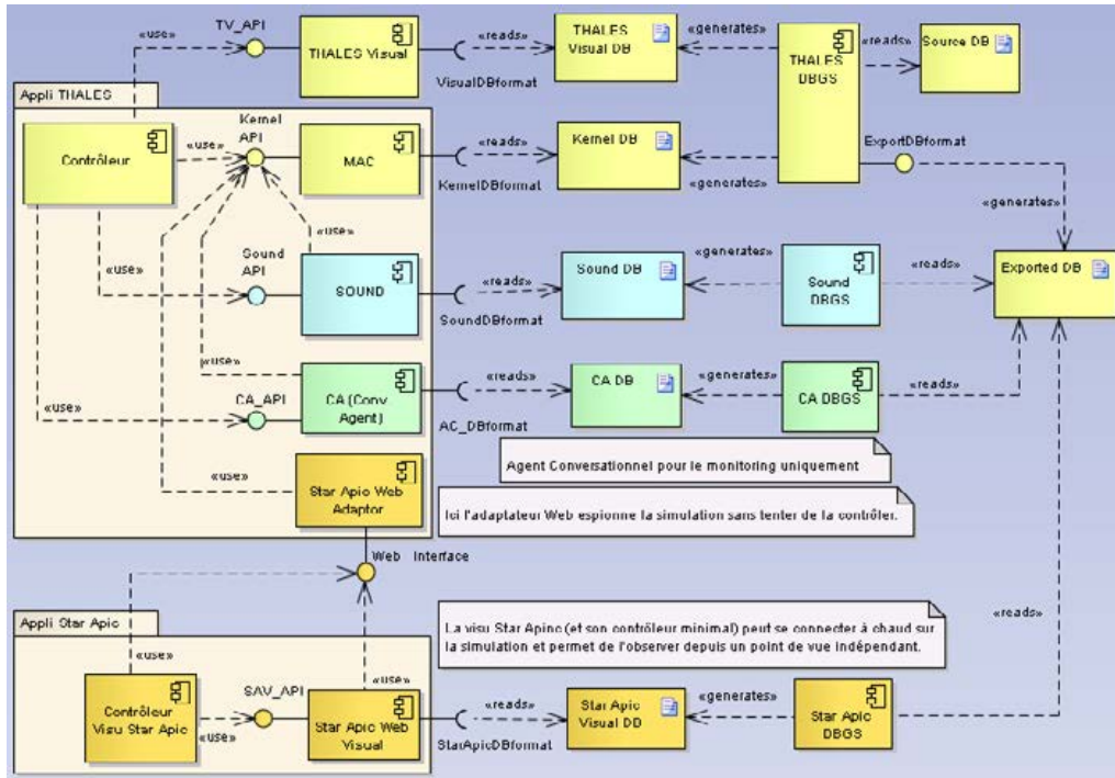
FIGURE 4.3 – Schéma de la structure globale du Projet Terra Dynamica
