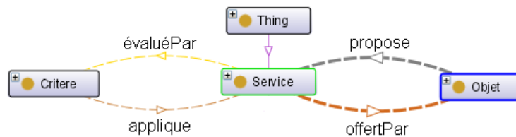
FIGURE 3.3 – Concepts généraux de l'ontologie de services «Niveau méta».
