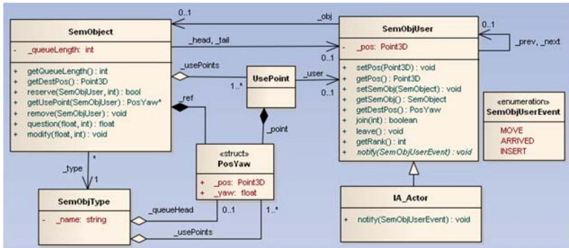
FIGURE 4.9 – Le diagramme de classes UML de la description d'un objet sémantique
