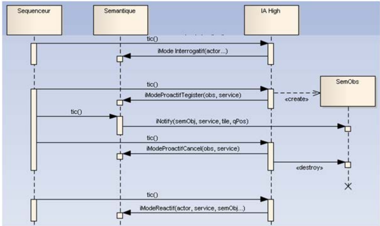
FIGURE 4.7 – Interactions entre le module sémantique et l'IA
