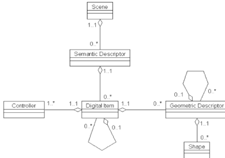
FIGURE 2.4 – Modèle sémantique XML-based de l'environnement virtuel autour de l' Item Digital , proposé dans [Gutierrez et al., 2005]
