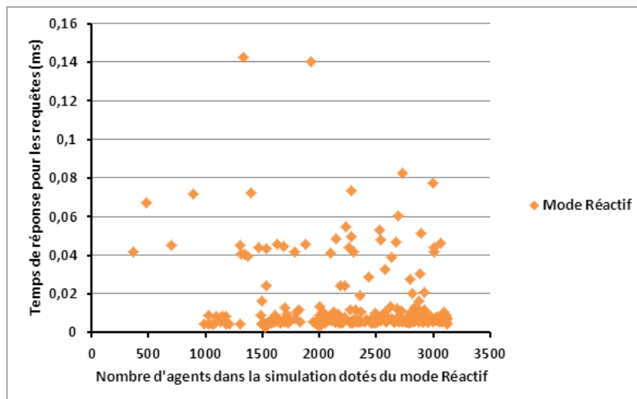
FIGURE 4.12 – Temps de réponse moyen pour les requêtes envoyées en Mode Réactif
