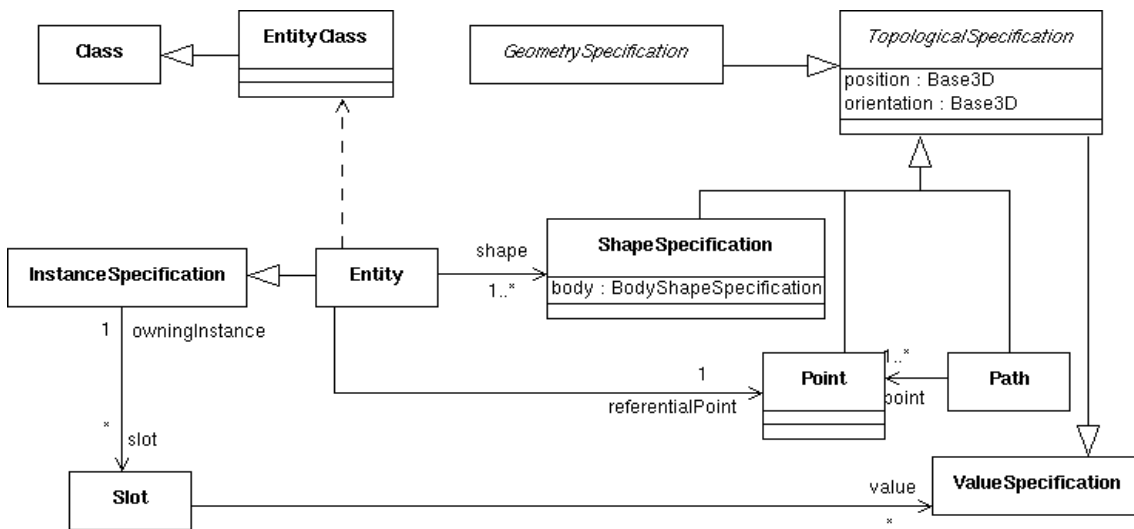
FIGURE 2.1 – Méta-modèle pour la modélisation des concepts du domaine dans Mascaret [Chevaillier et al., 2009]
