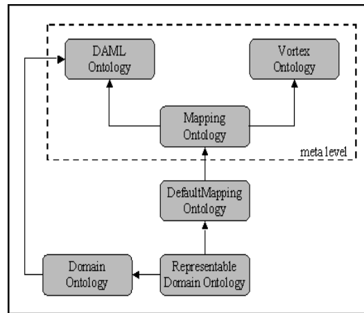
FIGURE 2.2 – Lien entre les différentes ontologies utilisées dans les travaux de [De Troyer et al., 2003]
