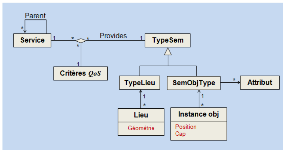
FIGURE 4.8 – Représentation des objets et lieux de l’environnement
