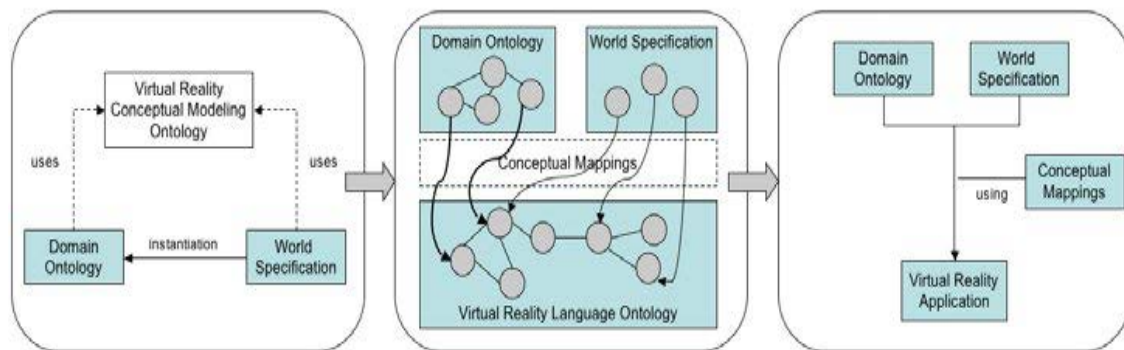
FIGURE 2.3 – Processus conceptuel VR-Wise proposé dans [Pellens et al., 2005] (de gauche à droite) : étape de spécification, étape de mapping et étape de génération
