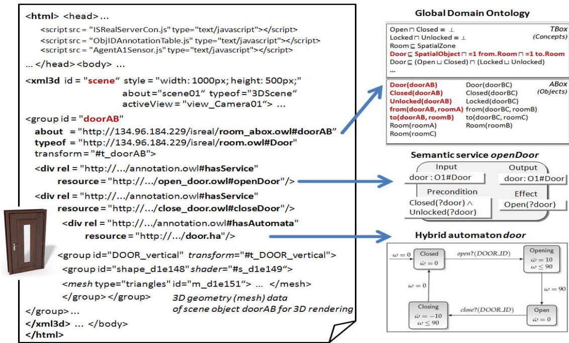
FIGURE 2.10 – Exemple d’annotation sémantique d’un objet graphique XML3D avec RDFa.
