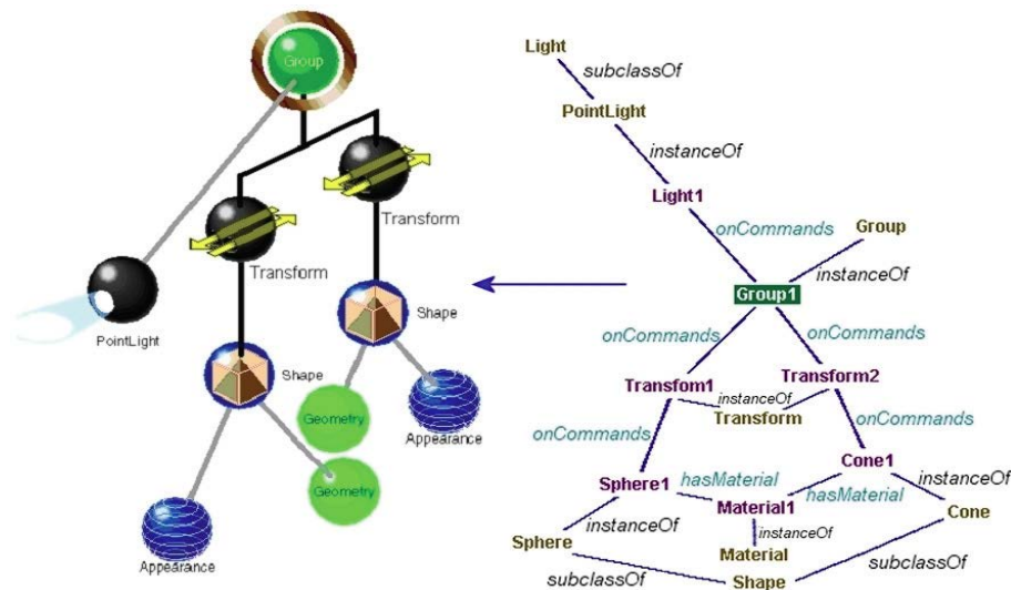
FIGURE 2.7 – Graphe OWL décrivant une scène dans [Kalogerakis et al., 2006]
