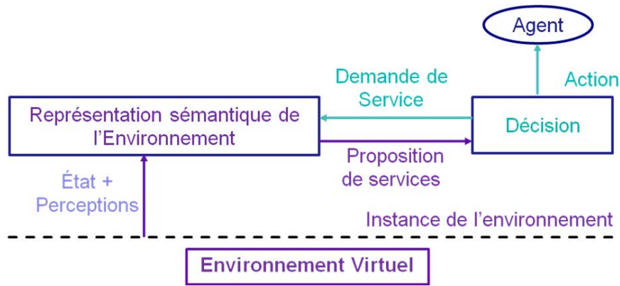
FIGURE 3.1 – Interactions du module sémantique de l'EV avec le module décisionnel des agents : le module décisionnel envoie des requêtes pour trouver un objet qui propose le service recherché, et le module sémantique lui renvoie une liste d'objets triés selon la QoS qu'ils proposent.
