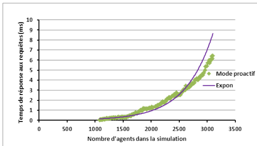
FIGURE 4.13 – Temps de réponse moyen pour les requêtes envoyées en Mode Pro-actif
