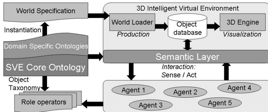
FIGURE 2.5 – Architecture de l'EV sémantique basée sur les ontologies proposée dans [Grimaldo et al., 2006a]
