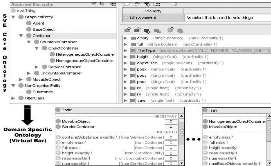
FIGURE 2.6 – Exemple de l'ontologie de domaine utilisée dans [Grimaldo et al., 2008]
