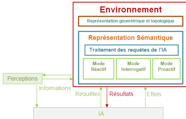
FIGURE 4.6 – Diagramme présentant les interactions du module sémantique de l’environnement avec les autres modules du projet
