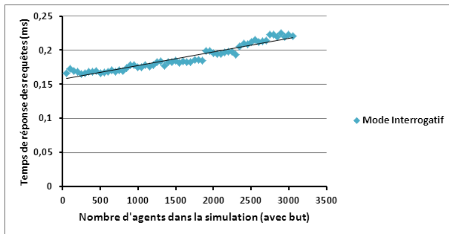
FIGURE 4.10 – Temps de réponse moyens aux requêtes du module d’IA par nombre d’agents
