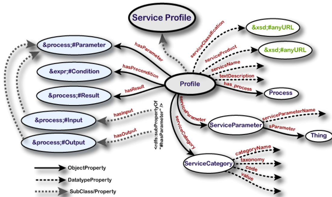
FIGURE 2.12 – Classe ServiceProfile de l'ontologie OWL-S
