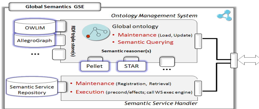
FIGURE 2.11 – Architecture du modèle sémantique de l’environnement virtuel de la plateforme ISReal proposée dans [Kapahnke et al., 2010]
