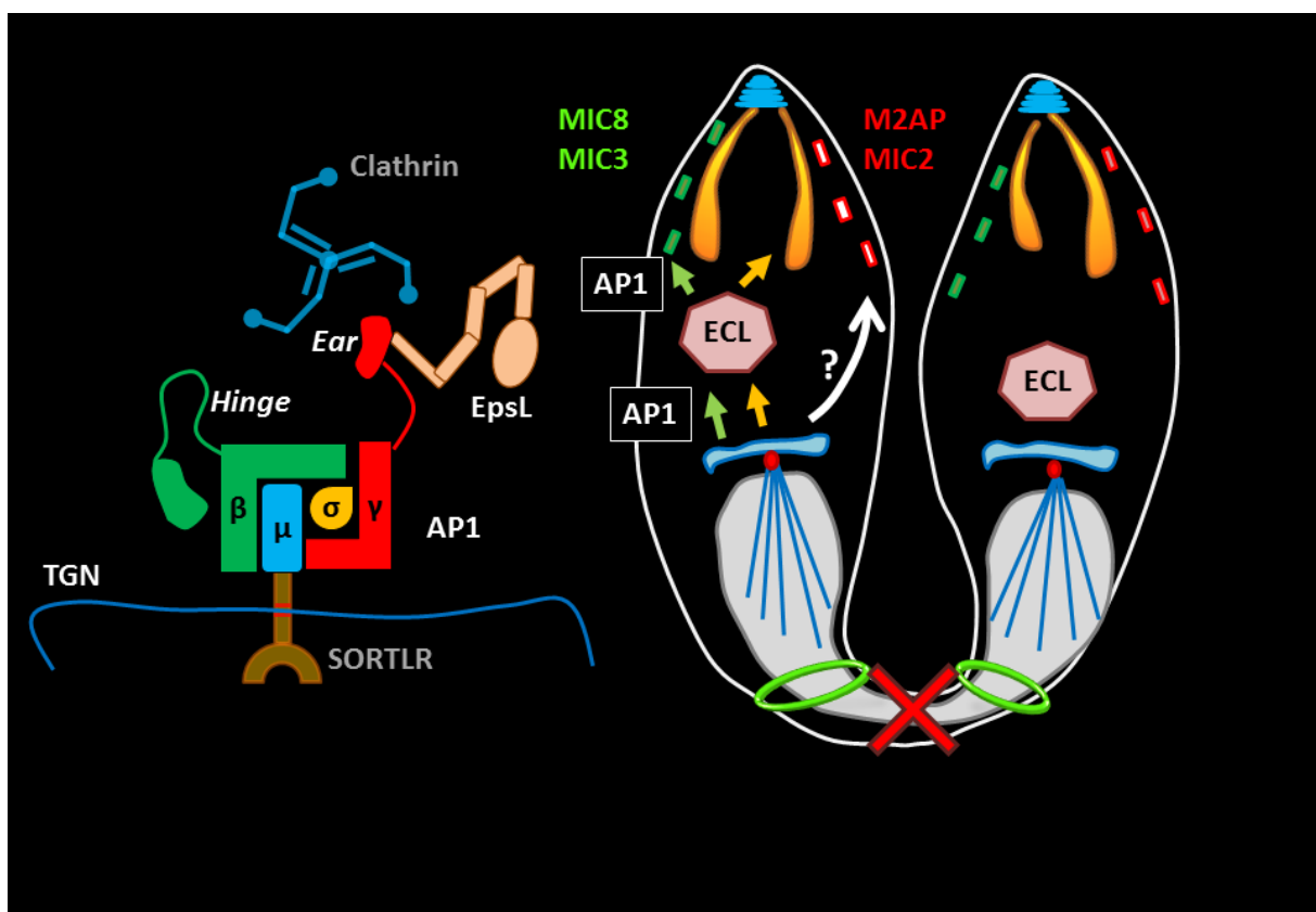
Figure 2 : Gauche : Modèle moléculaire du complexe fonctionnel de transport impliquant AP1. AP1 interagit avec le récepteur TgSORTLR par son domaine de reconnaissance du motif DiLeucine présent dans la queue cytoplasmique de TgSORTLR. AP1 recrute la clathrine par les domaines « Hinge » des sous-unités beta et gamma, et la protéine TgEpsL par le domaine « ear » de la sous-unité gamma. Ce
