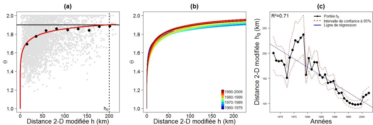
263 264 Figure 3 : Chutes de neige. (a) Fonction extrémale pour la première fenêtre d'estimation (1958-1977) : estimations du coefficient 265 extrémal pour chaque paires de stations (points gris), moyennes par classes de distance (points noirs) et fonction extrémale de 266 Brown-Resnick ajustée sur les estimations par paires (courbe rouge). La portée de la dépendance extrémale h_0 est égale à 200 km. 267 (b) Evolution temporelle de la fonction extrémale de Brown-Resnick, des fenêtres d'estimation les plus anciennes (en bleu) 268 jusqu'aux plus récentes (en rouge). (c) Evolution temporelle de la portée de la dépendance extrémale. L'axe des abscisses indique 269 le centre de la fenêtre d'estimation. L'intervalle de confiance à 95% est calculé par la méthode delta.
