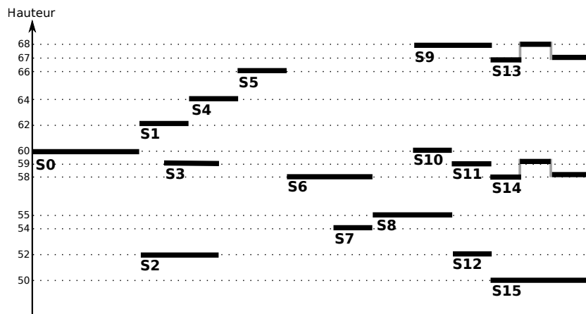
FIGURE 2.29 – Les fragments des contigs de l'algorithme CW peuvent être considérés comme des streams.
