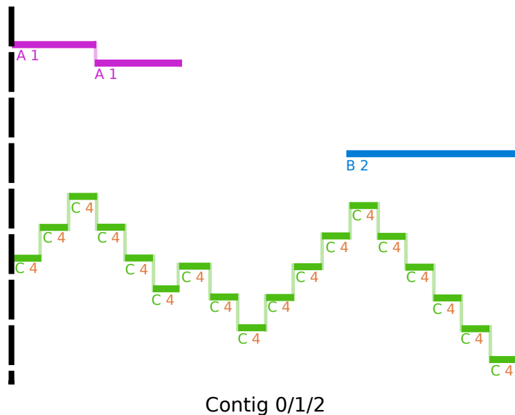
FIGURE 3.3 – Les notes des voix A et B ont été prédites correctement (3 Vrais Positifs), l'ensemble des notes de la voix C ont été prédites dans la voix 4 au lieu de la voix 3 (18 Faux Négatifs). AVC = (100\% + 100\% + 0\%)/3 = 66\% ; NPR = 3/21 = 14\% .
