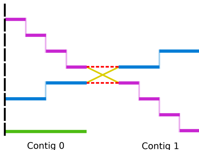
FIGURE 4.4 – Croisement de voix. Les précédentes méthodes de connexion commettaient une erreur (en pointillé ), en utilisant uniquement les valeurs des hauteurs pour connecter les fragments. En utilisant la moyenne des durées de l'ensemble des notes des fragments nous trouvons la bonne connexion à faire ( trait plein ).
