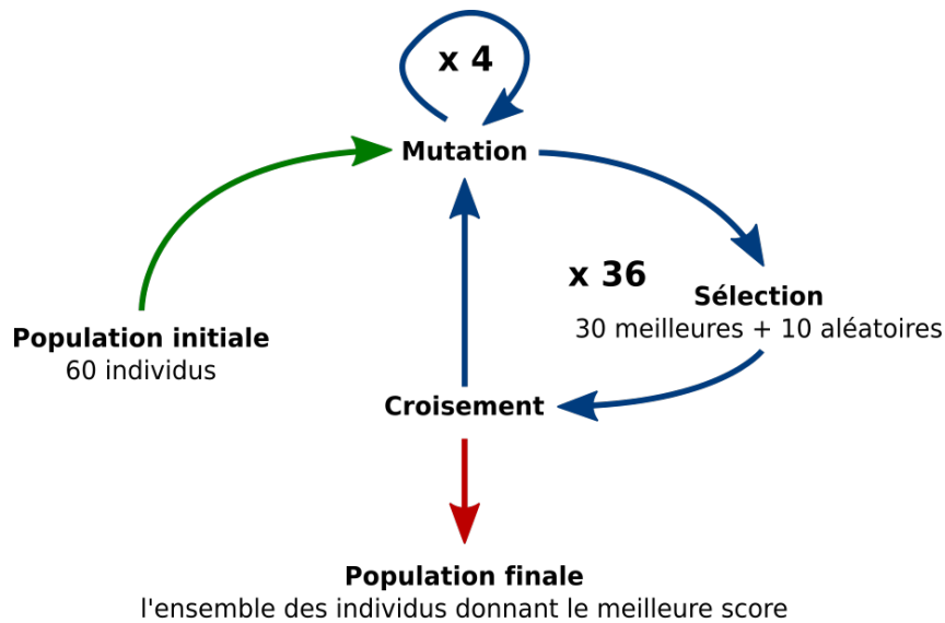
FIGURE 4.5 – Étapes principales de notre algorithme génétique.
