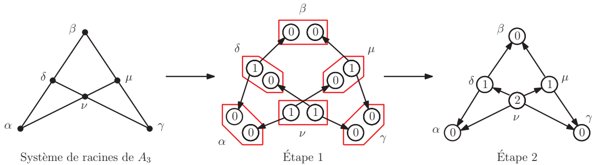
FIGURE 1.10. Construction d'un graphe valué bien assemblé sur un système de racine de A_3 . On peut vérifier que le treillis obtenu est bien isomorphe à (A_3, \leq_R) . Voir le chapitre 4 pour plus de détails sur cette construction.
