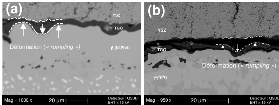
Figure 4. 28 : Dommages pouvant être attribués à une déformation de l'interface (« Rumpling ») pour un dépôt SPS YSZ sur AM1 revêtu \beta -(Ni,Pt)Al (a) et Pt- \gamma ' (b) après cyclage thermique
