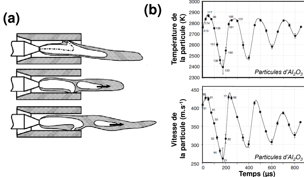
Figure 1. 27 : Jet plasma en mode claquage réamorçage [131] (a) et effet sur le traitement de particules d' Al_2O_3 en APS – adapté de [133] (b)
