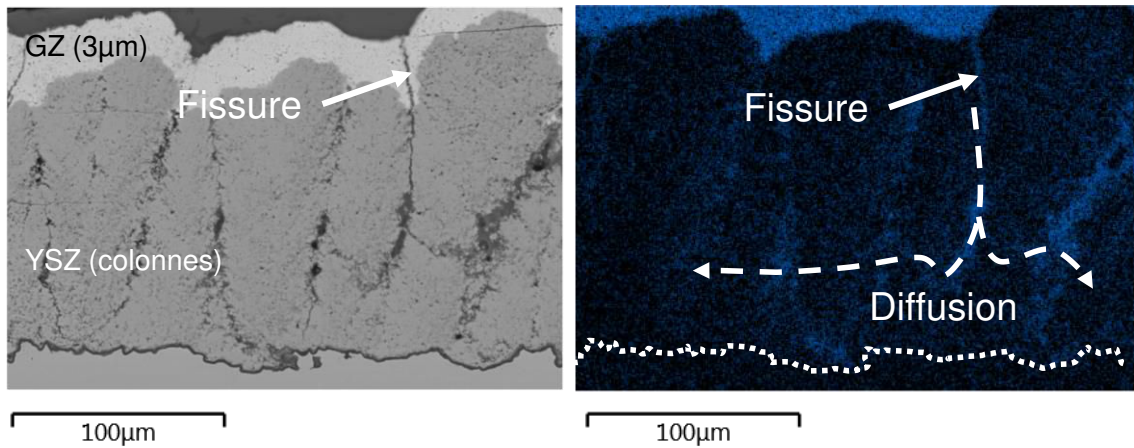
Figure 5. 29 : Réaction entre le CAS et le revêtement GZ observée après l'infiltration CAS4. À gauche, observations micrographiques MEB et à droite, clichés EDS du Calcium
