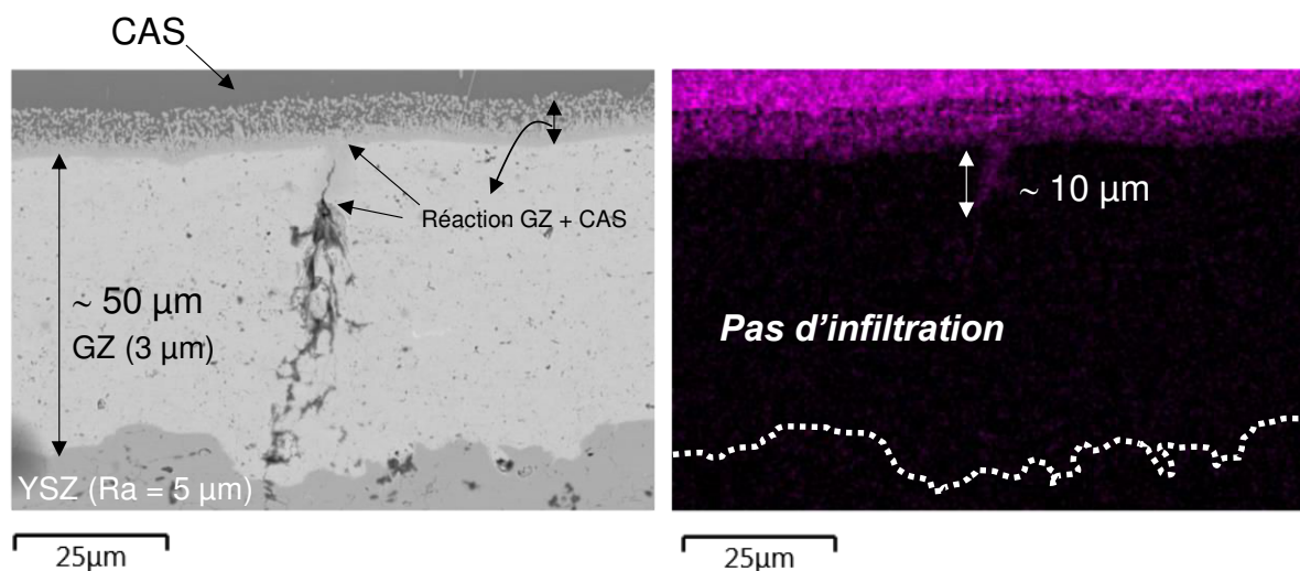
Figure 5. 21 : Zone fissurée obtenue après infiltration CAS de 1h à 1300 °C sur un dépôt réalisé avec la condition (16) et la suspension GZ/3 EIOH (Micrographie MEB à gauche) et cartographie EDS du silicium (à droite)
