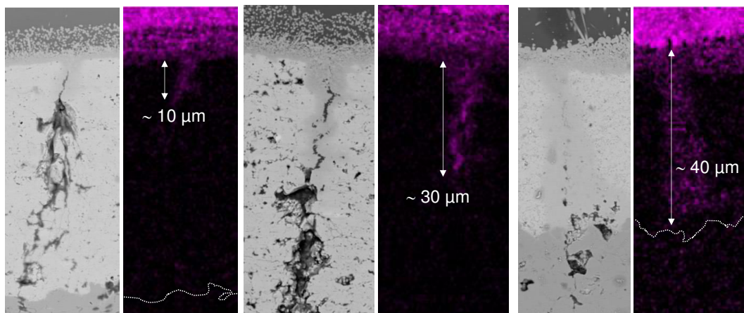
Réaction entre un contaminant de type CMAS et des dépôts \text{Gd}_2\text{Zr}_2\text{O}_7 obtenus par SPS
