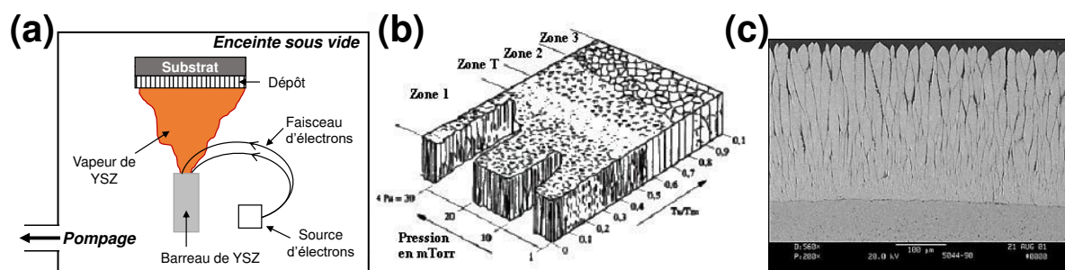
Figure 1. 6 : Schéma du procédé EB-PVD (a), diagramme de Thornton décrivant les dépôts obtenus [32] (b) et dépôt colonnaire YSZ (type zone 1) - image issue de [18] (c)
