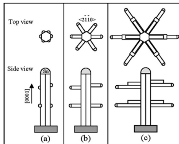
Figure I.8. Mécanisme de croissance des nano-hélices [30].
