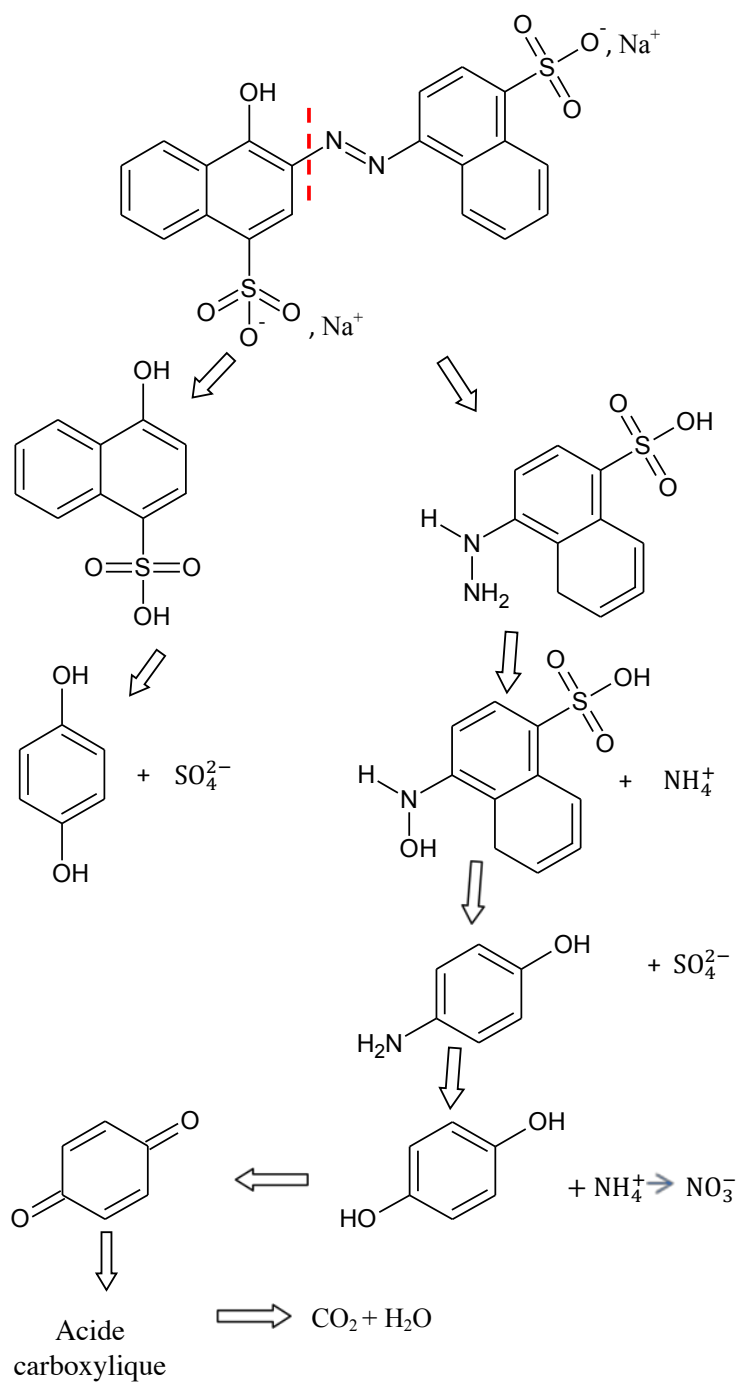
Figure IV.7. Mécanisme proposé pour la dégradation du colorant organique AR14.
