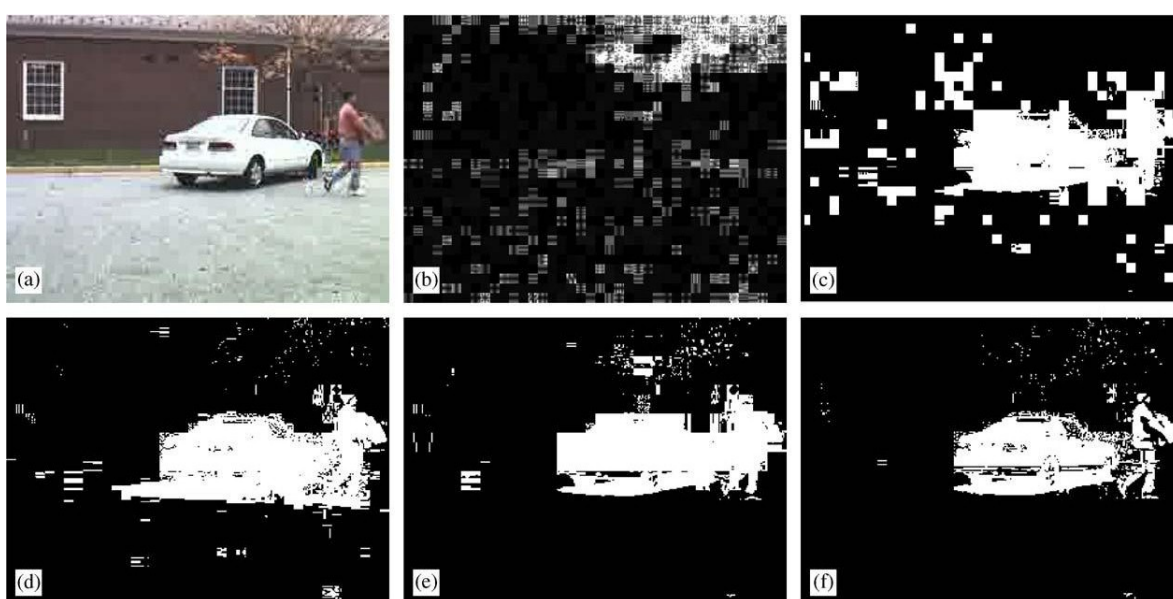
FIGURE 2.4 – Résultats de la détection de divers algorithmes basées sur la modélisation de l'arrière plan. [9] (a) image original, (b) déviations standard, (c) Horprasert et al. [41], (d) Stauffer et al. [36], (e) Elgammal et al. [40], (f) Kim et al. [9]
