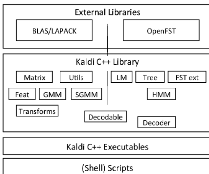
FIGURE 6.1 – Architecture de la boîte à outils Kaldi.
