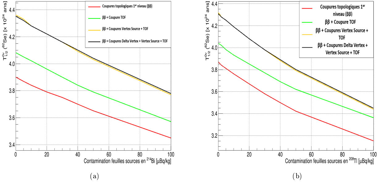
FIGURE 6.13: Evolution de la sensibilité du démonstrateur en fonction de la contamination en 214 Bi (a) et 208 Tl (b) des feuilles sources pour les coupures topologiques de 1 er niveau ainsi que les trois coupures adaptées à la rejection du radon. Le taux de radon considéré est de 150 µBq/m 3 et le calcul de sensibilité est obtenu à partir de la méthode ROI.
