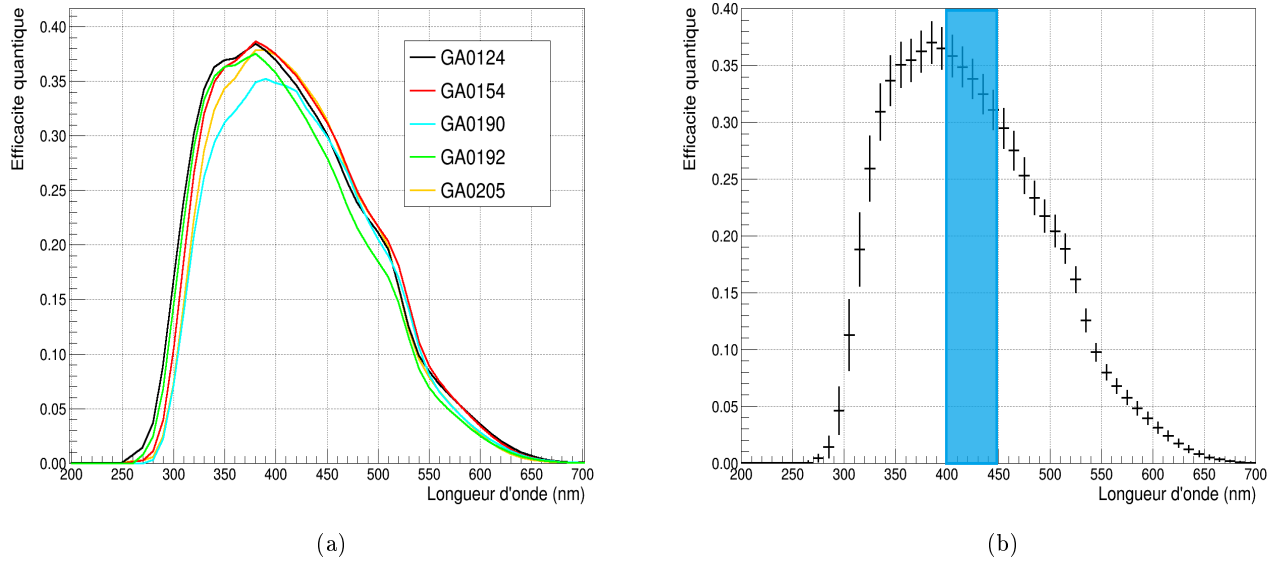
FIGURE 4.8: Efficacité quantique des cinq PMs 5'' de SuperNEMO utilisés pour la validation du modèle optique (a) et efficacité quantique moyenne calculée à partir des informations obtenues pour 19 des PMs 8'' de SuperNEMO en relation avec la zone du spectre d'émission du scintillateur (b). L'incertitude sur chaque point correspond à la largeur à 1\sigma de la distribution de l'efficacité quantique.
