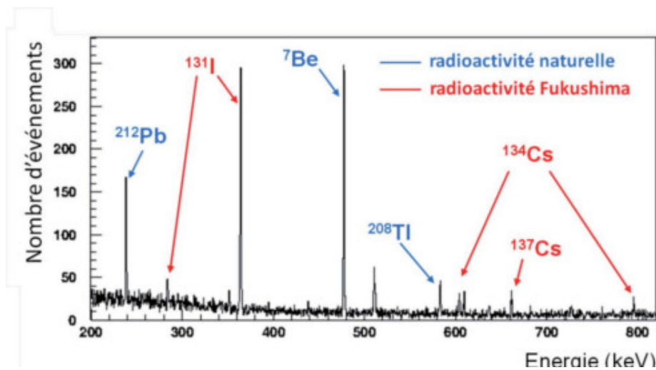
FIGURE 2.12: Illustration de la détermination des contaminations radioactives présentes dans un matériau par spectrométrie gamma. Chaque raie positionnée à une énergie donnée est représentative d'un isotope contenu dans l'échantillon.
