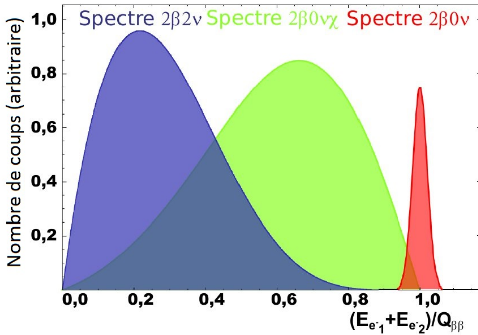
FIGURE 1.13: Représentation schématique de la somme de l'énergie des deux électrons émis ( E_{e_1} et E_{e_2} ) lors des décroissances double bêta avec émission de neutrinos, sans émission de neutrinos et dans le cas d'une émission d'une autre particule telle que le Majoron \chi . Q_{\beta\beta} représente l'énergie de transition.
