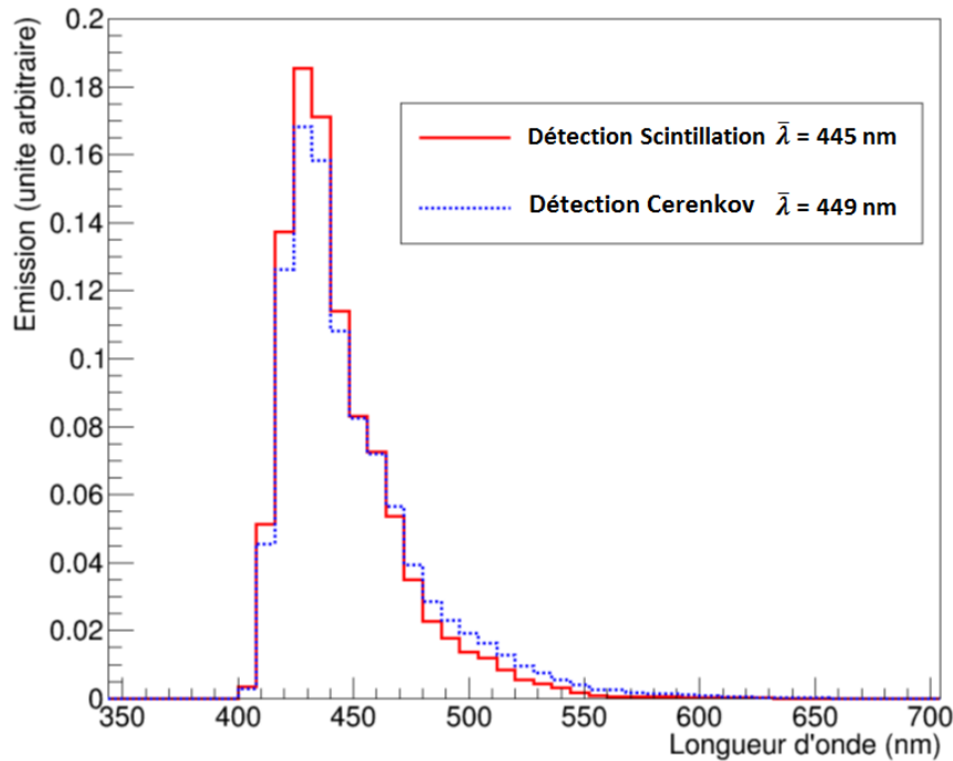
FIGURE 5.9: Spectres en longueurs d'onde simulés des photons détectés de scintillation et des photons issus du rayonnement Cerenkov pour un électron de 1 MeV interagissant au centre de la face avant du scintillateur.
