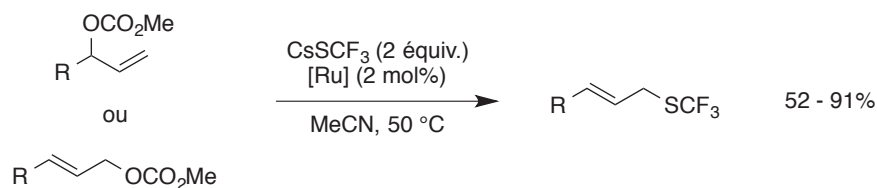
Schéma 40 : Utilisation du \text{CsSCF}_3
