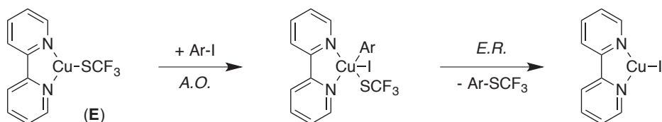
Schéma 86 : Addition oxydante / Elimination réductrice
