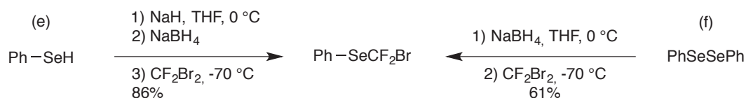
Schéma 113 : Bromodifluorométhylation de dérivés séléniés
