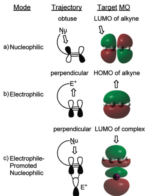
Figure 16 : HOMO/LUMO de différentes cyclisations intramoléculaires [457]
