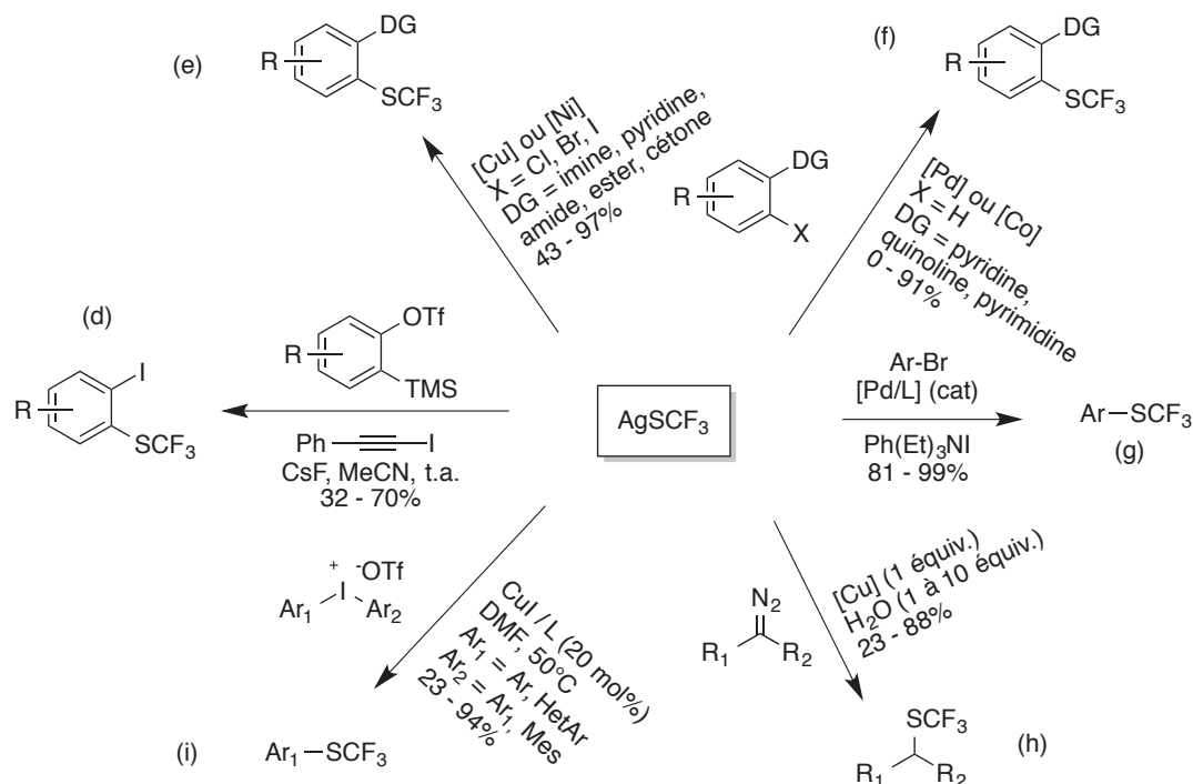
Schéma 32 : Nouvelles utilisations de \text{AgSCF}_3
