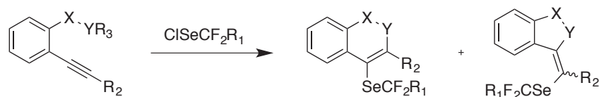
Schéma 154 : Formation de cycles à 6 chaînons
