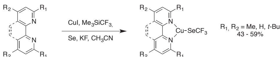
Schéma 124 : Synthèses de complexes de trifluorométhylsélénocuisse stables à l'air
