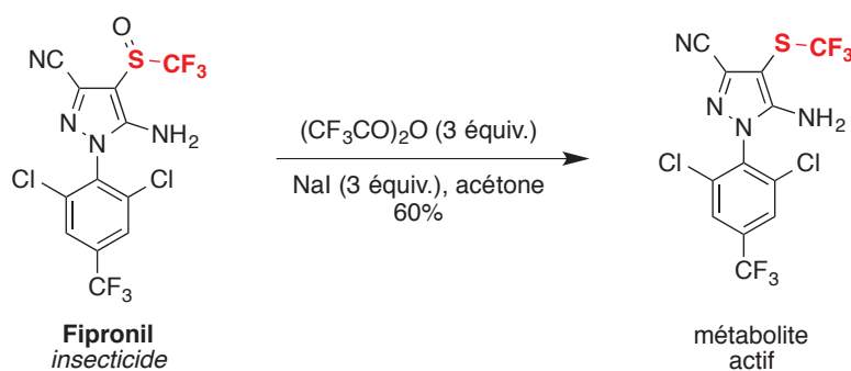
Schéma 18 : Réduction du Fipronil
