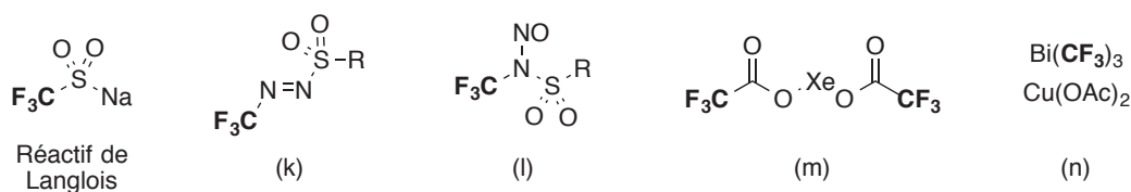
Figure 6 : Autres réactifs de trifluorométhylation radicalaire
