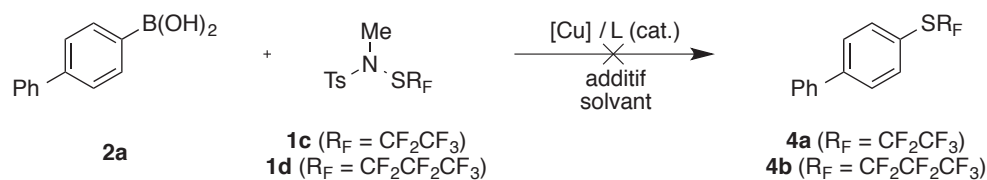
Schéma 84 : Extension aux analogues perfluorés
