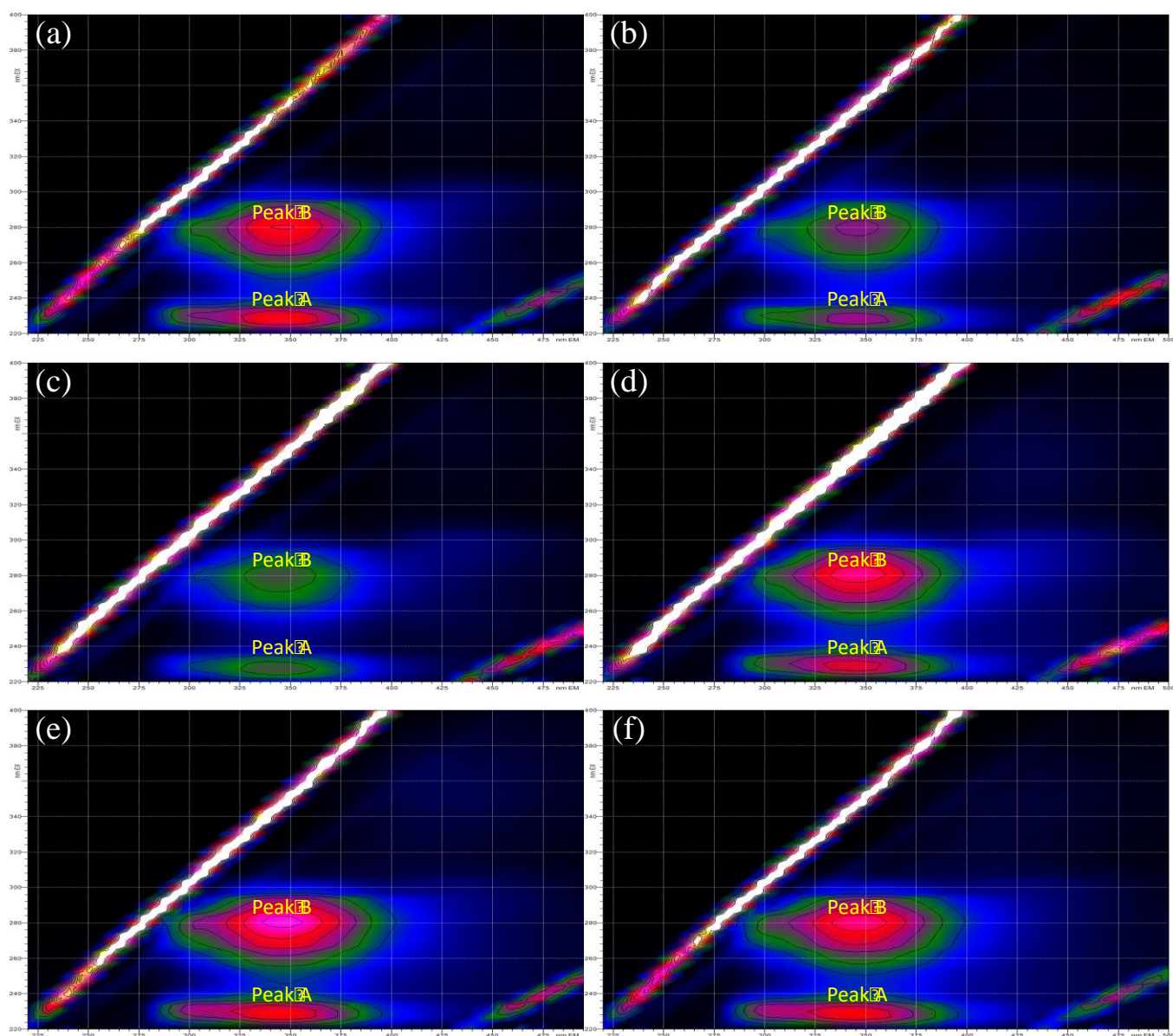
Fig. 5.6 EEM spectra of the EPS extracted from the fungus exposed to sub-toxic Ni 2+ concentrations: (a) 0 mg/L (dilution (d) 1/2), (b) 0.5 mg/L (d 2/5), (c) 1 mg/L (d 3/10), (d) 5 mg/L (d 4/5), (e) 10 mg/L (d 4/5), and (f) 25 mg/L (d 1/2).
