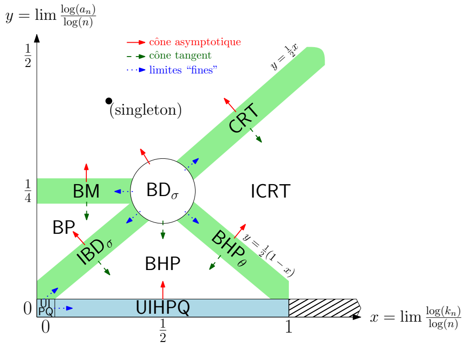
FIGURE 2.9 : La classification des limites de (V(Q_n^{k_n}), a_n^{-1} \cdot d_{gr}^{Q_n^{k_n}}, \rho_n) , avec Q_n^{k_n} une quadrangulation à n faces internes de périmètre 2k_n uniforme (d'origine \rho_n ), et a_n un facteur de renormalisation. (En fonction de x = \log(k_n)/\log(n) et y = \log(a_n)/\log(n) .)
