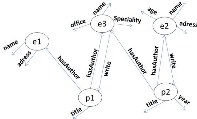
FIGURE 2.2 – Exemple d'un graphe de données
