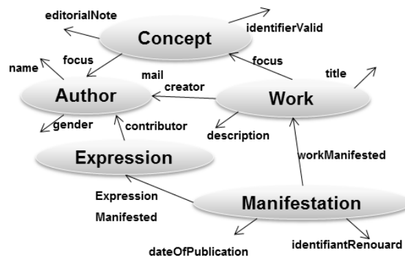
FIGURE 6.2 – Le schéma déclaré dans le jeu de données de la figure 6.1.
