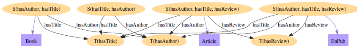
FIGURE 2.29 – Schéma extrait à partir des données du graphe G [10].
