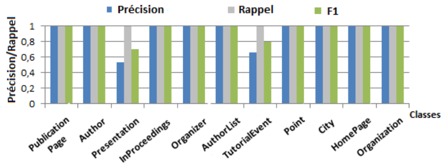
FIGURE 3.20 – Qualité des types attribués aux nouvelles entités du jeu de données Conference .
