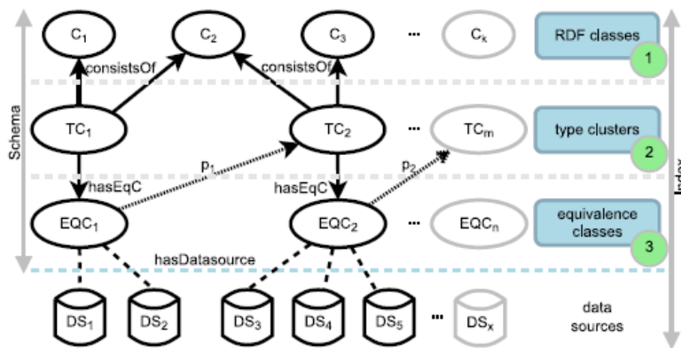
FIGURE 2.25 – Structure de l'index renforcée avec deux couches supplémentaires tirant parti des déclarations rdf:type [8]
