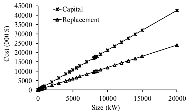
Figure 28. Evolution du prix avec la taille du générateur photovoltaïque
