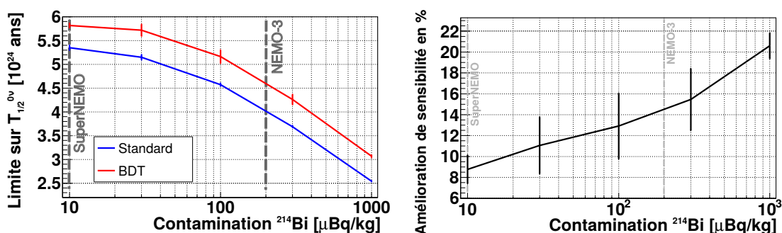
Figure 8.24 – (gauche) Évolution de la sensibilité du démonstrateur en fonction de la contamination 214 Bi pour les approches univarié (en bleu) et multivariée (en rouge). (droite) Amélioration sur la sensibilité apportée par l'utilisation d'une analyse multivariée en fonction de la contamination 214 Bi.
