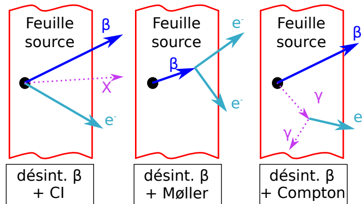
Figure 8.12 – Principaux mécanismes de production d'évènements de bruit de fond interne ( i.e. provenant de la source).
