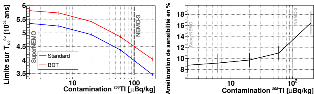
Figure 8.23 – (gauche) Évolution de la sensibilité du démonstrateur en fonction de la contamination 208 Tl pour les approches univarié (en bleu) et multivariée (en rouge). (droite) Amélioration sur la sensibilité apportée par l'utilisation d'une analyse multivariée en fonction de la contamination 208 Tl.
