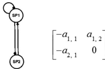
Figure VI-2: Exemple d'un graphique directionnel et de la matrice de communauté associée entre les populations de deux espèces (SP1 et SP2).
