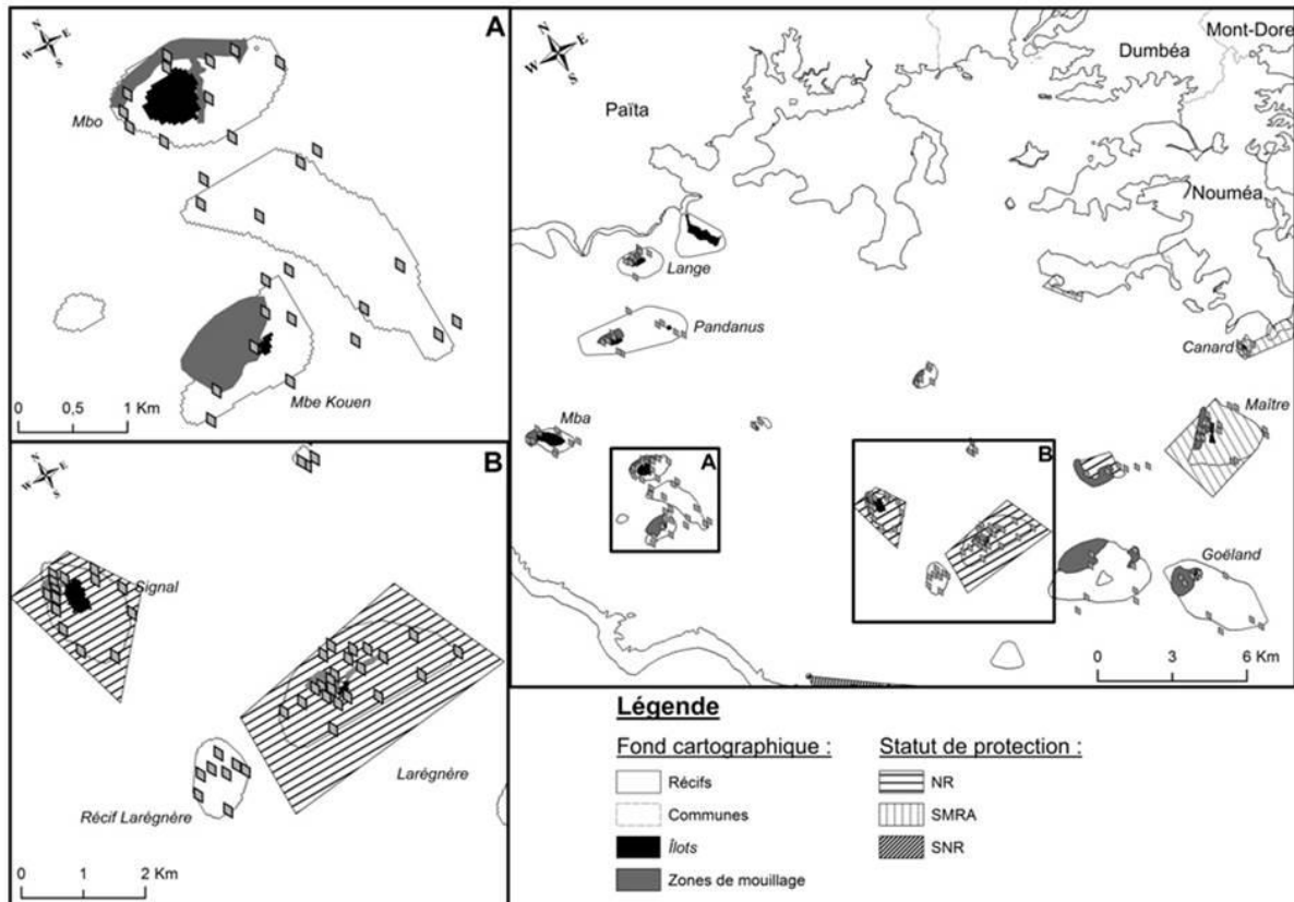
Figure V-2: Îlots et récifs du lagon du Grand Nouméa et positionnement des stations d'observation réalisées en 2013
