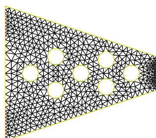
FIGURE 1.2 – Exemple de maillage d'une console en deux dimensions.
