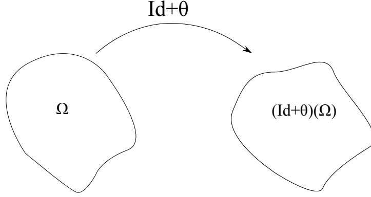
FIGURE 1.1 – Transformation du domaine \Omega par le difféomorphisme Id + \theta .
