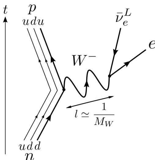
FIGURE 5.3 : Description de la désintégration \beta^- d'un neutron en proton, par l'émission d'un boson virtuel W^- qui se désintègre en un électron et un anti-neutrino (modification d'une figure issue de wikipédia). Les chiralités des quarks et de l'électron n'ont pas été indiquées, ces particules ayant des termes de masse après brisure de symétrie causant une oscillation entre les deux états de chiralité lors de leur propagation.
