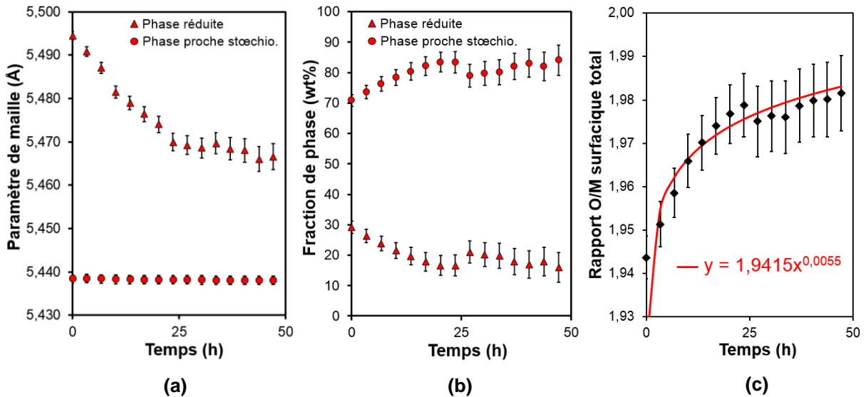
Figure 55. Evolution (a) des paramètres de maille, (b) des fractions de phase et (c) du rapport O/M surfacique total à T_{amb} au sein de l'oxyde mixte U_{0,55}Pu_{0,45}O_{2-x} exposé à N_2 + \sim 30 vpm O_2 + \sim 50 vpm H_2O .
