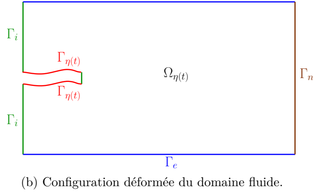
FIGURE 3 – Configurations du domaine fluide (chapitres 2, 3 et 4)
