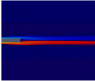
FIGURE 4 – Vorticité de l'écoulement stationnaire à Reynolds 200.
