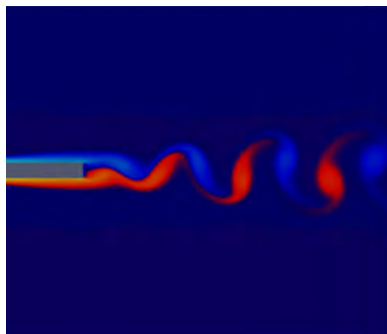
FIGURE 5 – Vorticité de l'écoulement perturbé.
