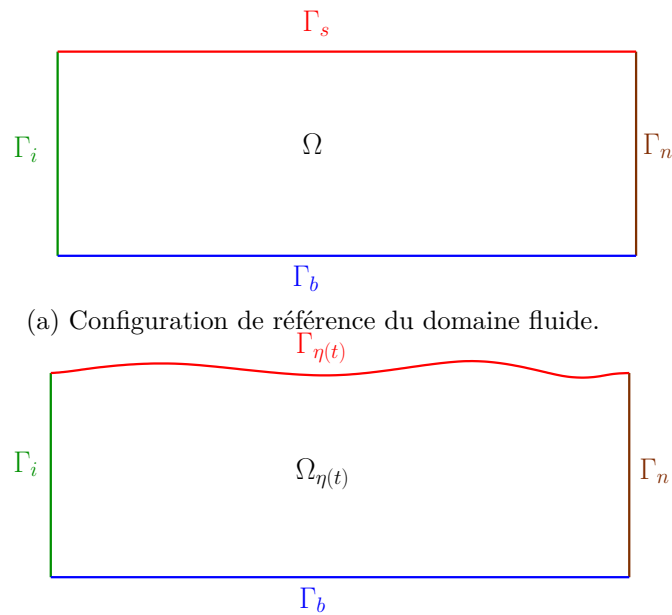
(b) Configuration déformée du domaine fluide.
