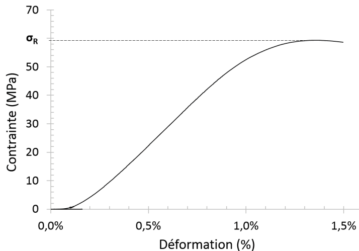
FIGURE 2.17 – Courbe contrainte-déformation pour un échantillon de pin laricio ( \sigma_r = 59.3 \text{ MPa} )
