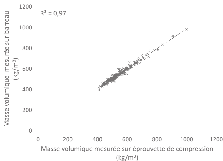
FIGURE 2.33 – Masse volumique ( kg/m^3 ) des éprouvettes barreaux en fonction de la masse volumique ( kg/m^3 ) des éprouvettes de compression correspondantes
