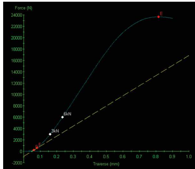
FIGURE 2.16 – Exemple de courbe de force en fonction du déplacement pour un échantillon de pin laricio ( \sigma_r = 59.3 \text{ MPa} )
