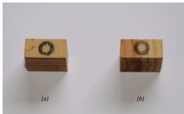
FIGURE 2.18 – Exemples de repères circulaires réalisés à l'encre sur une face du plan TL (a) et une face du plan RL (b), de chaque éprouvette
