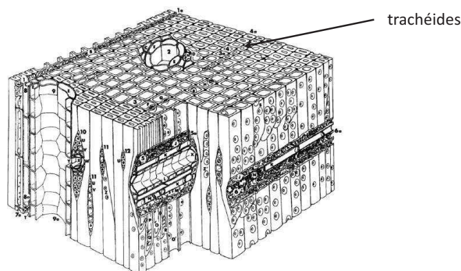
FIGURE 1.4 – Diagramme schématique d'un bloc de bois de pin d'après Howard et Manwiller, dans Siau (1984)
