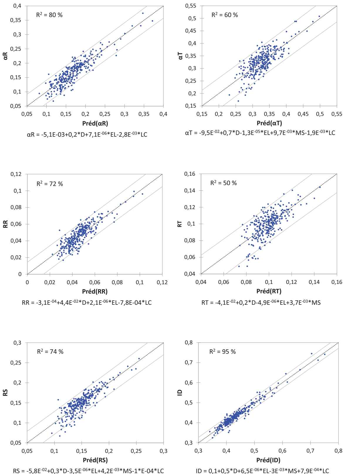
FIGURE 3.16 – Représentation graphique des régressions des variables issues des mesures hygrosopiques en fonction de leur valeur prédite par le modèle
