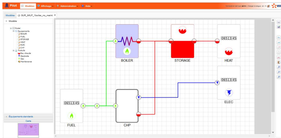
FIGURE 3.14 – Modèle PILOT (PLNE) de l'installation de cogénération
