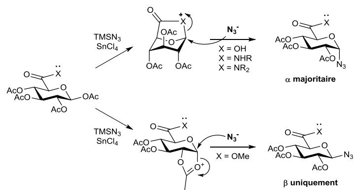
Schéma 33 – Synthèse d'acides et d'esters 1-azido-6-glucuroniques.
