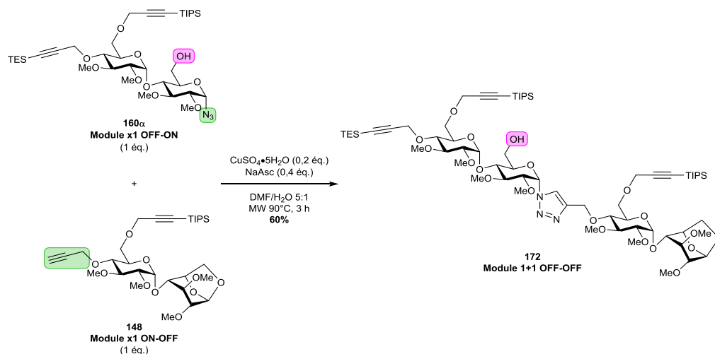
Schéma 92 – Synthèse du module 1+1 OFF-OFF .
