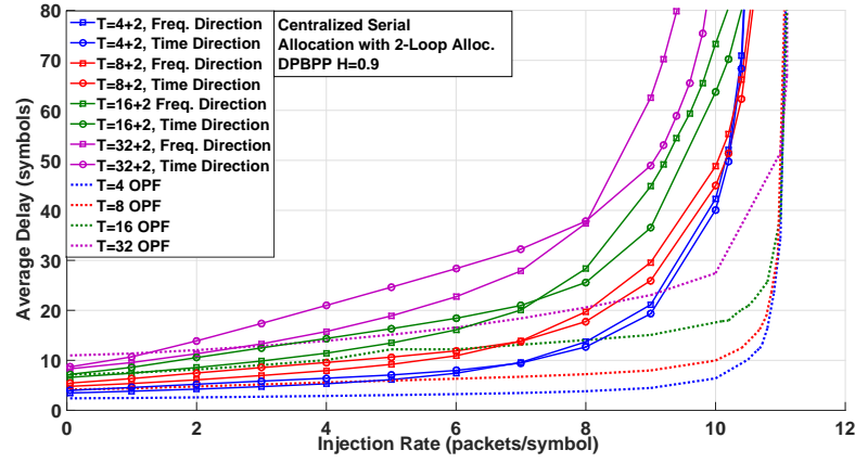
FIGURE 0.11: Latence moyenne en fonction de l'augmentation du taux d'injection pour un trafic réaliste non-uniforme (DPBPP) pour l'allocation série (2 iterations) avec l'approche centralisée pour différentes longueurs de trame.
