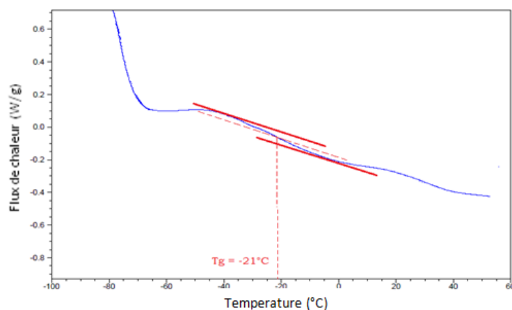
Figure 3.3: Courbe DSC réalisée sur un échantillon de "polyisoprène+amorceur thermique" réticulé à 120^\circ\text{C}
