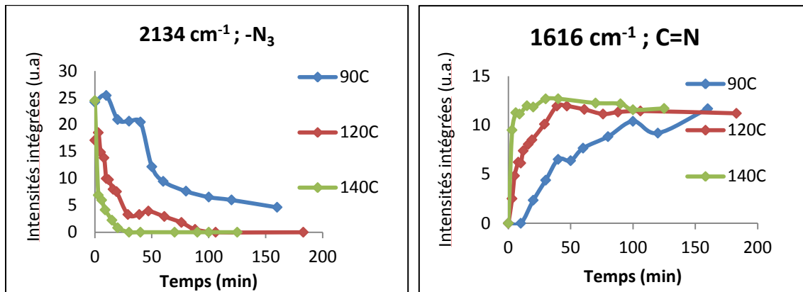
Figure 2.24: Evolution des bandes centrées à 2134 et 1610 \text{cm}^{-1} en fonction de la température de chauffage
