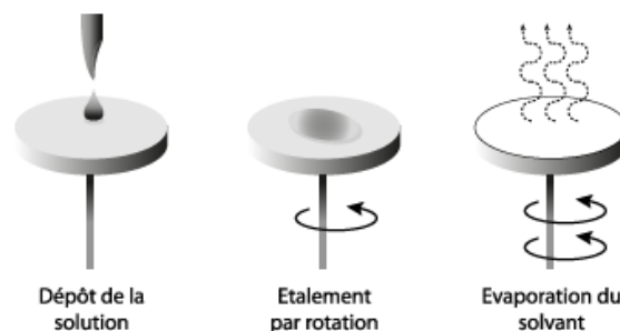
Figure 1.23: Représentation schématique du procédé de dépôt de couche mince par spin coating
