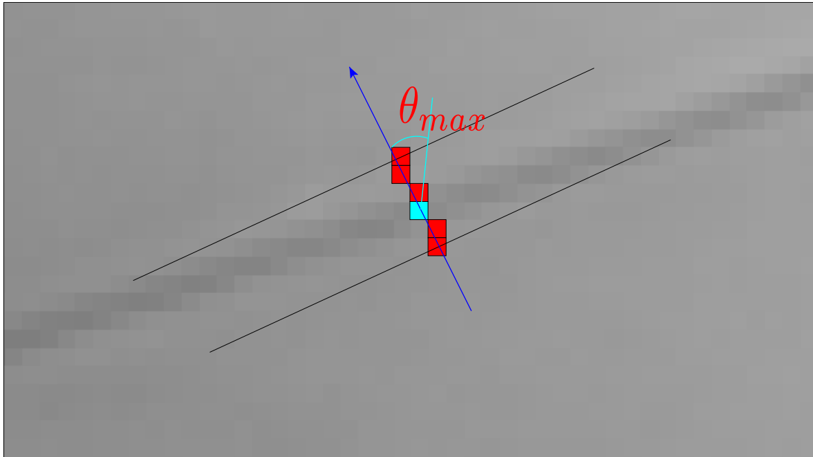
FIGURE 3.6 – Illustration de la sélection d'un pixel sur un segment de droite ayant le gradient le plus fort et dont l'angle entre la direction de parcours et la direction du gradient est inférieur au seuil \theta_{max} = \{\frac{\pi}{2}, \frac{\pi}{8}, \frac{\pi}{10}\} (Les auteurs précisent que se sont des valeurs empiriques validées sur des images réelles).
