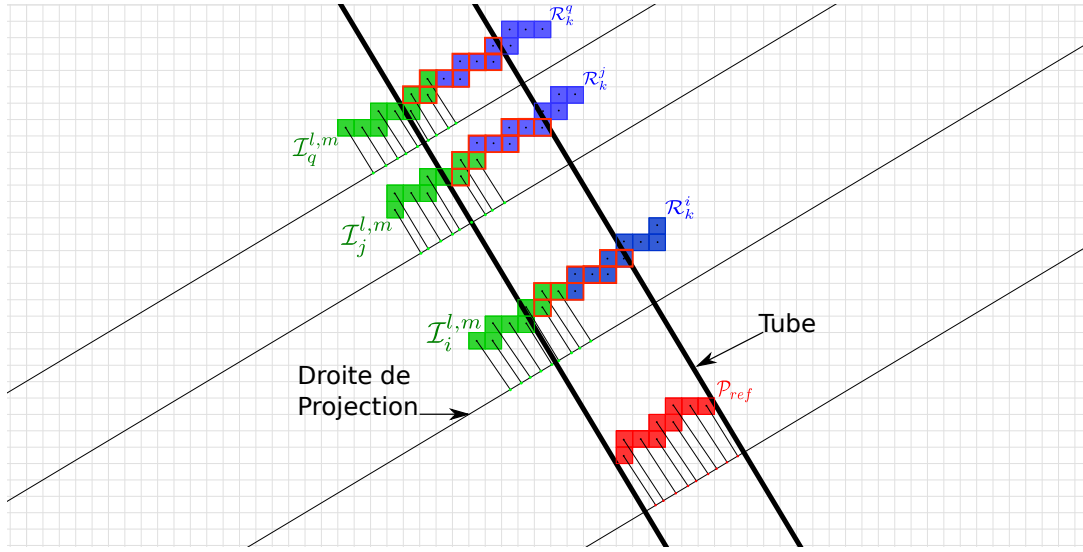
FIGURE 4.17 – Illustration utilisée pour l'étude de l'algorithme avec interpolation.
