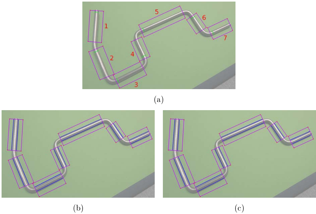
FIGURE 5.4 – Résultats de l’algorithme sur le modèle « fond vert » — (a) Initialisation de l’algorithme — (b) version sans interpolation — (c) version avec interpolation.
