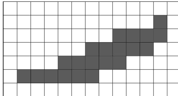
(e) segment épais D(3, 7, 0, 16)
