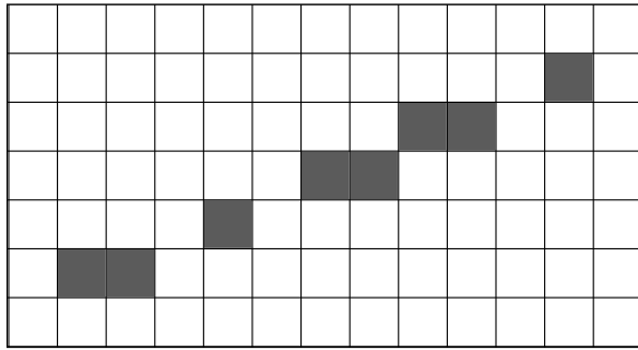
(a) segment déconnecté D(3, 7, 0, 5)
