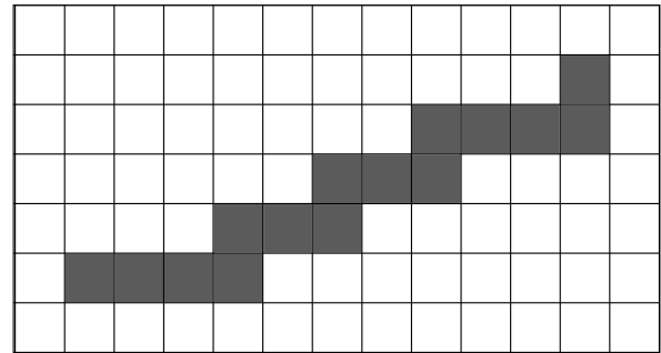
(d) segment standard D(3, 7, 0, 10)
