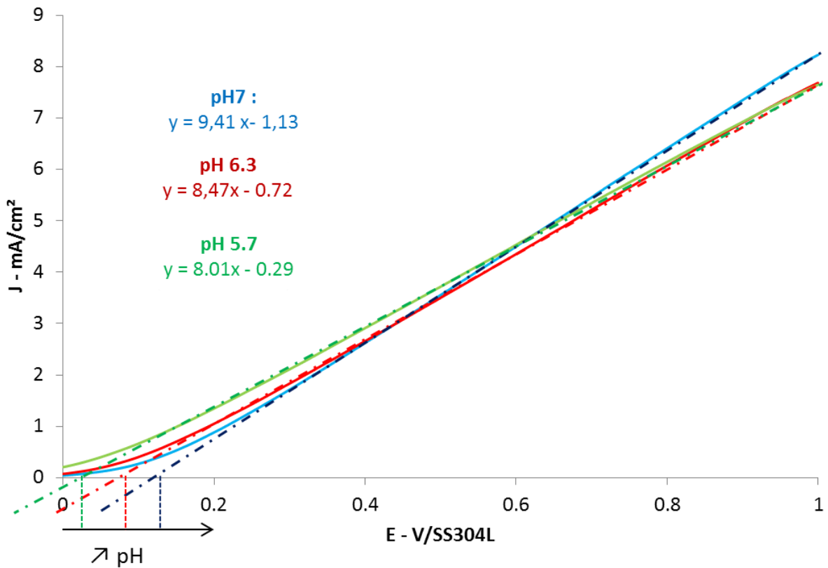
Figure 61 : Voltampérométrie de 1V à 0V/SS304L sur acier 304L dans 120 mmol.L -1 de NaCl et 10 mmol.L -1 de CBS (40% de sucre), à différents pH ; pH 7 : bleu ; pH 6.3 : rouge ; pH 5.7 : verte.
