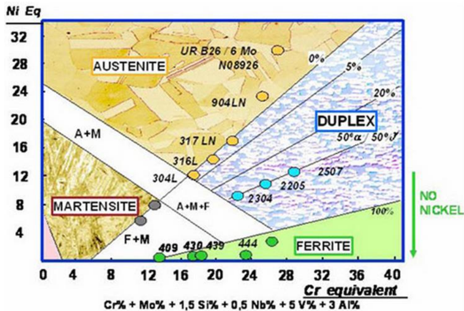
Figure 8 : Diagramme de Schaffer : famille d'aciers inoxydables (source : http://www.keytometals.com/ , Lean Duplex Stainless Steel ).
