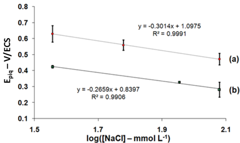
Figure 26 : Potentiel de piqûration ( E_{\text{piq}} ) en fonction du logarithme de la concentration en chlorure (a) AISI 304L, (b) AISI 430 (pH 7, 25 °C).
