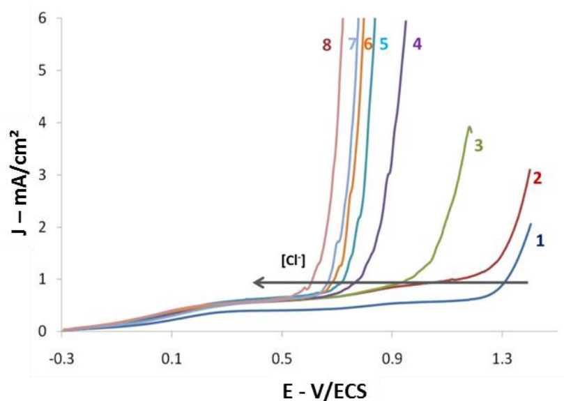
Figure 7 : Voltampérométries linéaires sur électrode d'acier inoxydable 304L en milieu tampon carbonate ( 36 \text{ mmol.L}^{-1} , \text{pH}=6,4 ) contenant différentes concentrations en NaCl (1 : 0 ; 2 : 20 ; 3 : 30 ; 4 : 45 ; 5 : 60 ; 6 : 75 ; 7 : 90 ; et 8 : 120 \text{mmol.L}^{-1} ) [18].
