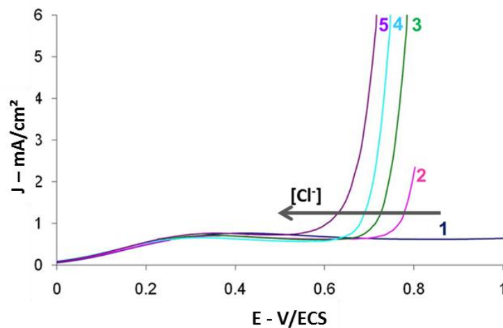
Figure 5 : Voltampérogrammes linéaires sur électrode de nickel en milieu tampon carbonate (CBS : 36 mmol.L -1 , pH=6.4) contenant différentes concentrations en NaCl (1 : 0 mmol.L -1 ; 2 :36 mmol.L -1 ; 3 :60 mmol.L -1 ; 4 :90 mmol.L -1 ; et 5 : 120 mmol.L -1 ) [14].
