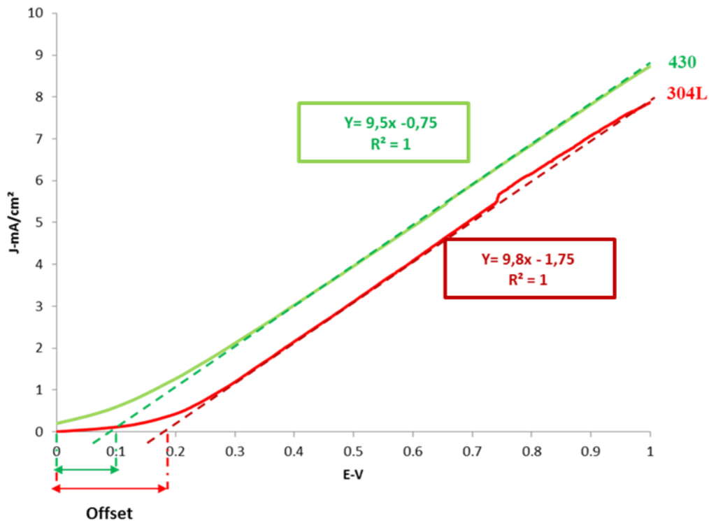
Figure 60 : Comparaison des courbes médianes de voltampérométries obtenues sur aciers inoxydables 304L (rouge) et 430 (verte) dans 120 mmol.L -1 de NaCl, 36 mmol.L -1 , pH 7, 40 %mq de saccharose.
