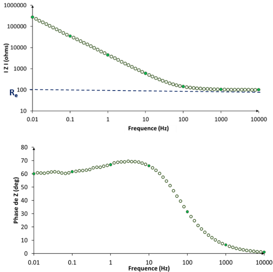
Figure 29 : Exemple d'un diagramme de Bode obtenu sur acier inoxydable 304L dans 120 \text{ mmol.L}^{-1} de NaCl à pH 7 : Détermination de la résistance d'électrolyte R_e .
