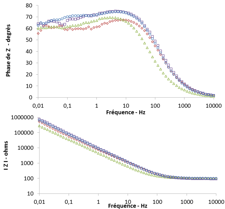
Figure 33 : Diagrammes de Bode obtenus dans une solution de NaCl à 120 \text{ mmol.L}^{-1} à pH 7 sur différents aciers inoxydables : 304L (triangles verts) ; 430 (ronds bleus) ; 430T (carrés violets) ; D2205 (losanges rouges).
