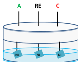
Figure 55 : Schéma du montage à trois électrodes A et C jouent alternativement le rôle d'électrode de travail et de contre électrode. L'électrolyte est une solution de 120 \text{ mmol.L}^{-1} de NaCl (pH 7 CBS 36 \text{ mmol.L}^{-1} ) contenant 40% m de saccharose.
