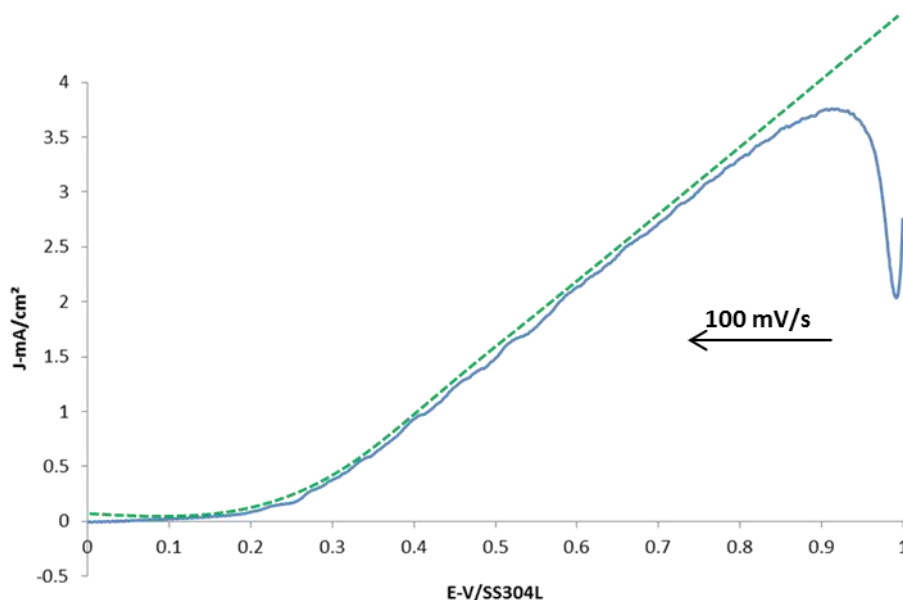
Figure 58 : Voltampérométrie cyclique à 100 \text{ mV.s}^{-1} dans 120 \text{ mmol.L}^{-1} de NaCl (pH 7) sur acier inoxydable 304L (bleue) ; courbe attendue (verte). Montage à trois électrodes en AISI 304L.
