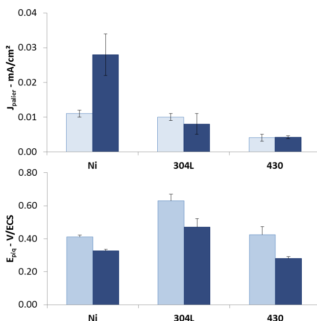
Figure 25 : Histogramme représentant la variation de J_{palier} et E_{piq} en fonction du matériau et de la concentration en ions chlorure ; bleu foncé : 120 \text{ mmol.L}^{-1} ; bleu clair : 36 \text{ mmol.L}^{-1} .
