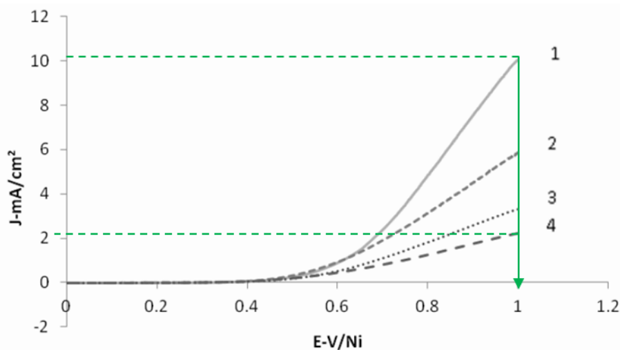
Figure 51 : Voltampérométrie de 1 V à 0 V/Ni (8 s) sur électrode de Ni dans une solution à 120 \text{ mmol.L}^{-1} de NaCl pH 7 ( 36 \text{ mmol.L}^{-1} CBS) avec 1 : 0% ; 2 : 30% ; 3 : 40% ; 4 : 50% de saccharose. (100 mV/s)
